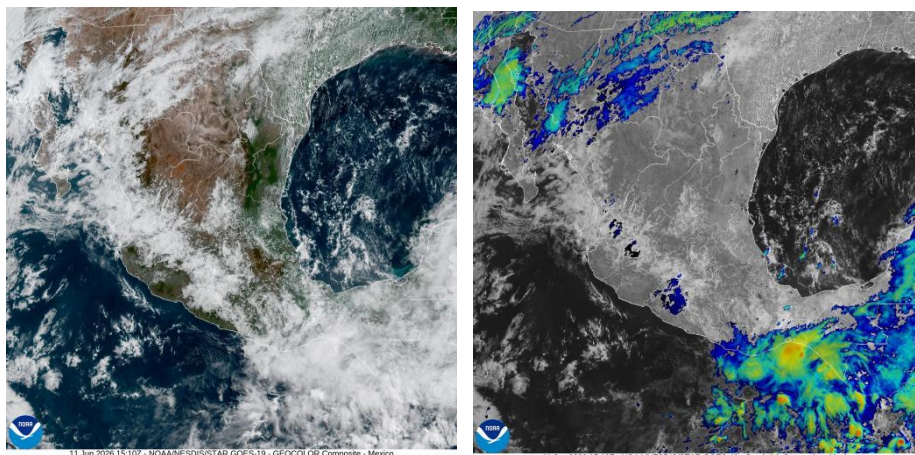
Figura 1. Imagen de satélite en canal luz visible (izquierda) e infrarrojo (derecha) obtenido del satélite GOES, 08:00 a.m. (hora local) del 11 de junio de 2026.
