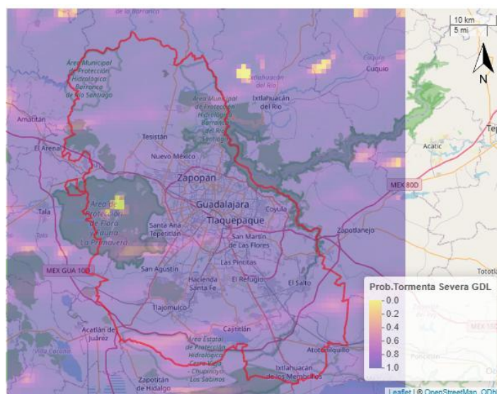
Figura 6: Pronóstico de desarrollo de tormentas para el 11 de junio de 2026. Consultado a las 09:00 a.m. (hora local) desde el modelo
