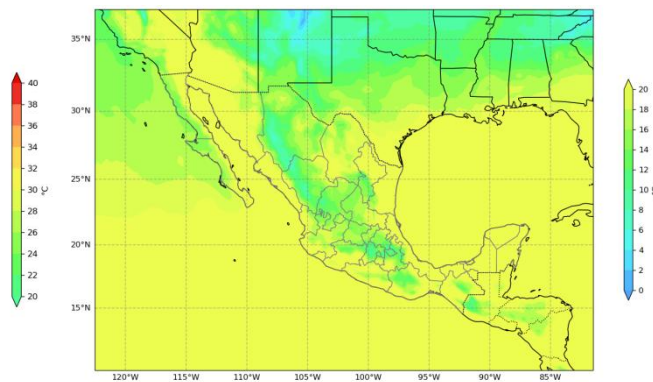
Figura 5: Temperatura mínima (°C) pronosticada a 24 horas. Modelo WRF (inicializado con GFS). Válido para el 13 de junio de 2026, 00 UTC.
