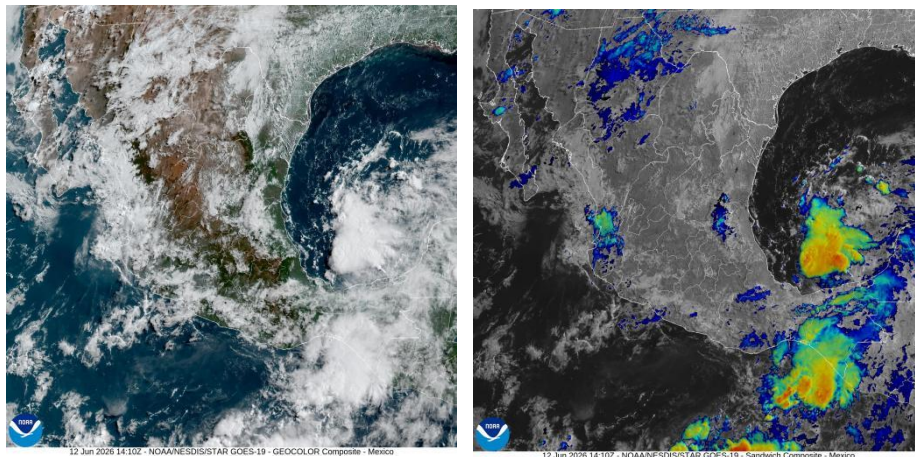
Figura 1. Imagen de satélite en canal luz visible (izquierda) e infrarrojo (derecha) obtenido del satélite GOES, 08:00 a.m. (hora local) del 12 de junio de 2026.
