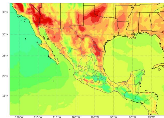
Figura 4: Temperatura máxima (°C) pronosticada a 24 horas. Modelo WRF (inicializado con GFS). Válido para el 13 de junio de 2026, 00 UTC.
