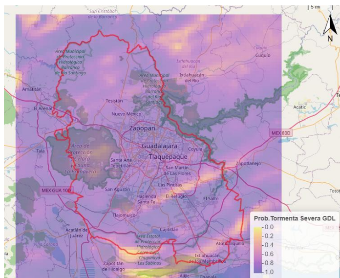
Figura 6: Pronóstico de desarrollo de tormentas para el 12 de junio de 2026. Consultado a las 09:00 a.m. (hora local) desde el modelo GFS.
