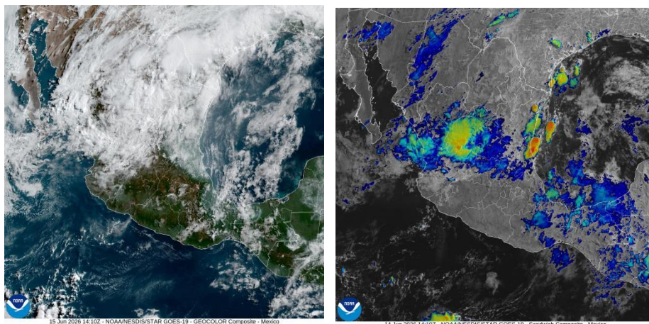
Figura 1. Imagen de satélite en canal luz visible (izquierda) e infrarrojo (derecha) obtenido del satélite GOES, 08:00 a.m. (hora local) del 15 de junio de 2026.
