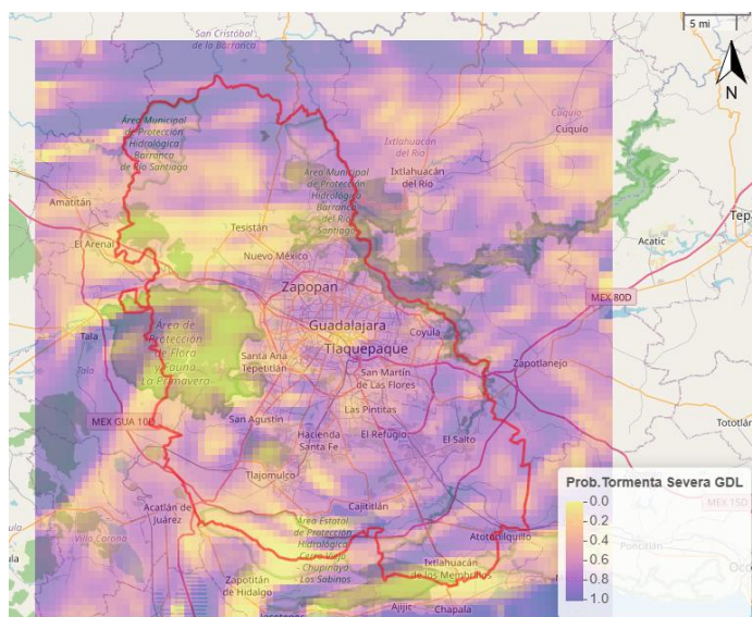
Figura 6: Pronóstico de desarrollo de tormentas para el 15 de junio de 2026. Consultado a las 09:00 a.m. (hora local) desde el modelo GFS.
