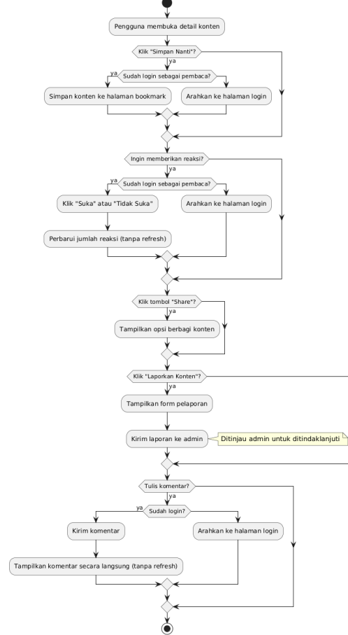
Activity Diagram - Interaksi Pengguna terhadap Konten
