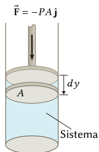
Figura 7.2: Um pistão que comprime uma quantidade de gás dentro de um recipiente cilíndrico exerce uma força de módulo PA . Quando um deslocamento dy do gás é considerado, podemos quantificar o trabalho realizado pelo pistão sobre o gás.
