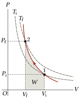
Figura 7.7: A curva 1 \rightarrow 2 representa uma compressão adiabática. Também são mostradas as isotermas correspondentes às temperaturas inicial e final do sistema.
