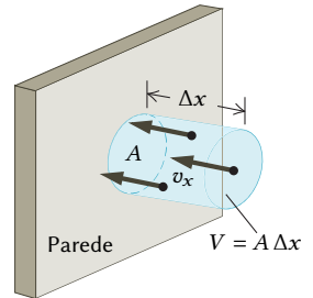
Figura 6.12: Elemento de volume de um gás.
