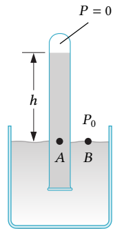
Figura 3.6: Barômetro de mercúrio.
