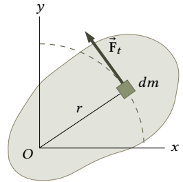
Figura 1.15: Um objeto rígido girando em torno de um eixo que passa através de O . Cada elemento de massa dm gira em torno de O com a mesma aceleração angular \alpha .
