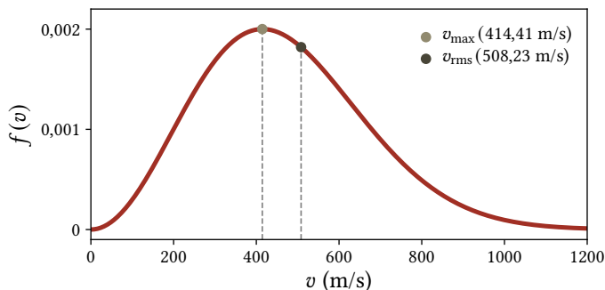
Figura 6.13: Distribuição de velocidade das moléculas do ar (seco) a 300 K (massa molar = 28,97 g/mol). A função f(v) se aproxima de zero quando v tende ao infinito.
