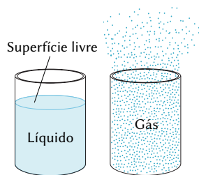
Figura 3.1: Ao contrário de um líquido, um gás não forma uma superfície livre e se expande para preencher todo o espaço disponível.
