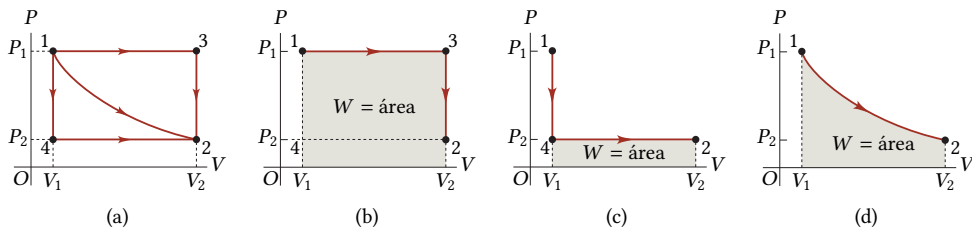
Figura 7.4: O trabalho realizado durante um processo para mudar um sistema de um estado inicial 1 para um estado final 2 depende do caminho escolhido para ir de 1 → 2.
