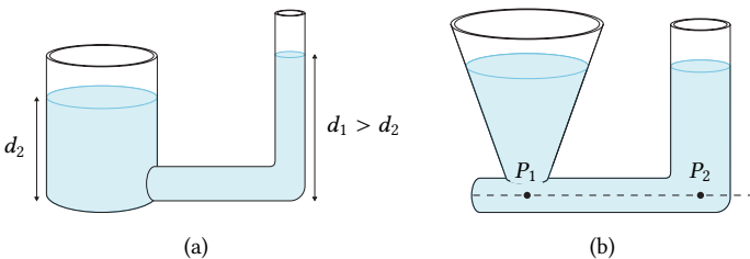
Figura 3.4: (a) Essa situação não pode ocorrer, já que pela condição de equilíbrio hidrostático, d_1 = d_2 . (b) Pela lei de Stevin, as pressões a uma mesma profundidade devem ser iguais, P_1 = P_2 .
