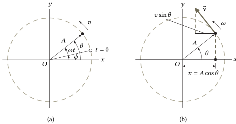
Figura 4.6: Uma partícula move-se em uma trajetória circular com velocidade constante v . (a) A componente x de sua posição descreve um movimento harmônico simples, e (b) a componente x de sua velocidade descreve a velocidade do movimento harmônico simples.
