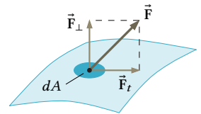
Figura 3.2: Força normal ( F_{\perp} ) e força tangencial ( F_t ) sobre a superfície de um elemento de fluido.
