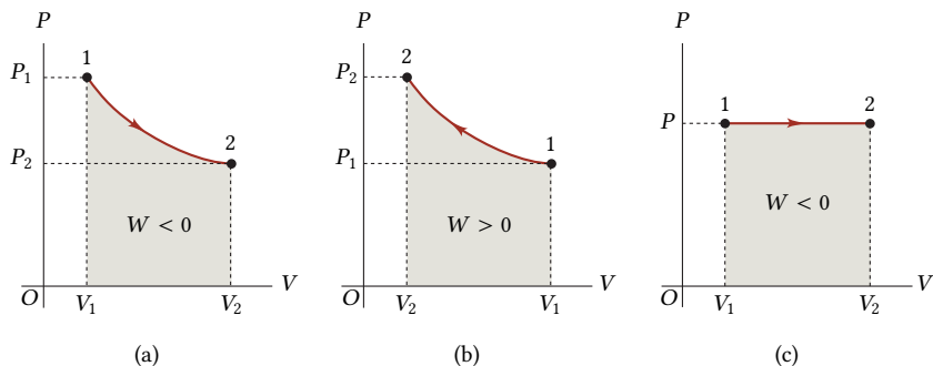
Figura 7.3: (a) O trabalho realizado sobre um sistema é negativo em uma expansão. (b) O oposto ocorre em uma compressão, já que a variação de volume é negativa e o trabalho, positivo. (c) Exemplo de uma expansão a pressão constante (isobárica).
