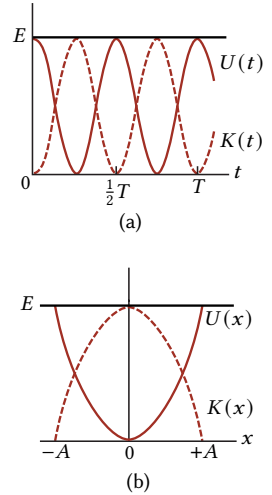
Figura 4.7: (a) Energia potencial U(t) , energia cinética K(t) e energia mecânica E como funções do tempo t para um oscilador harmônico linear. (b) Energia potencial U(x) , energia cinética K(x) e energia mecânica E como funções da posição x para um oscilador harmônico linear com amplitude A .
