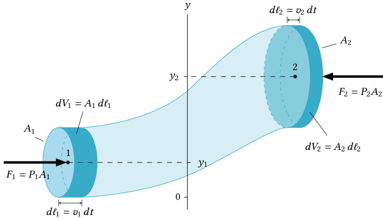
Figura 3.16: Tubo de corrente.
