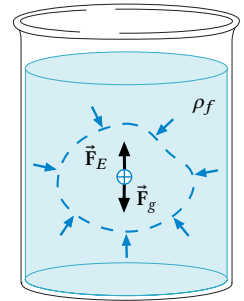
Figura 3.9: Diagrama de forças que atuam no elemento de volume: força de empuxo se iguala à força gravitacional no equilíbrio estático.
