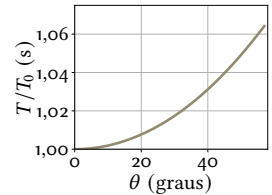
Figura 4.10: Período relativo em função da amplitude \theta .
