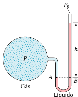
Figura 3.7: Manômetro de tubo aberto.
