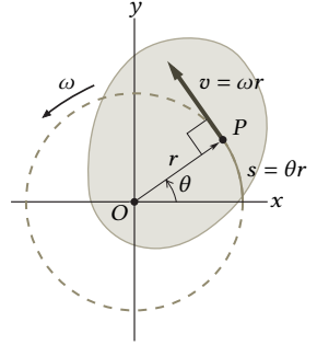
Figura 1.4: À medida que um corpo rígido gira em torno do eixo fixo através de O , o ponto P possui uma velocidade tangencial \vec{v} que está sempre tangente à trajetória circular de raio r .
