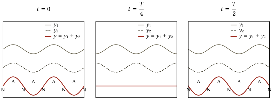
Figura 5.12: Padrões de ondas estacionárias produzidas em vários instantes de tempo por duas ondas de mesma amplitude viajando em direções opostas. Para a onda resultante, os nodos (N) são pontos de amplitude mínima/nula e os antinodos (A) são pontos de amplitude máxima.
