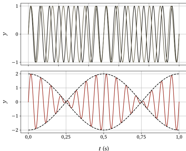
Figura 5.13: Batimentos são formados pela combinação de duas ondas com frequências aproximadamente iguais, neste caso de 14 e 16 Hz. Acima: as duas ondas individuais. Abaixo: a onda resultante; a linha tracejada representa o batimento de frequência igual a 2 Hz.
