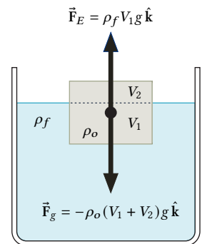
Figura 3.10: Forças que atuam sobre um objeto com volume V = V_1 + V_2 e densidade \rho_o que está flutuando em um fluido de densidade \rho_f .
