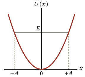
Figura 4.1: Função energia potencial U(x) = \frac{1}{2}kx^2 para valores positivos de k .
