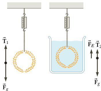
Figura 3.11: Quando a coroa está suspensa no ar, a escala mostra seu peso real porque T_1 = F_g . Quando a coroa é imersa na água, a força de empuxo \vec{F}_E altera a leitura da escala para um valor menor T_2 = F_g - F_E .
