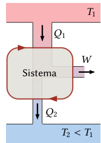
Figura 8.1: Máquina térmica.
