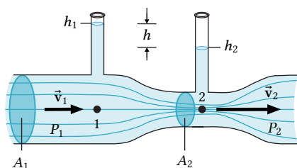
Figura 3.18: Medidor de Venturi.
