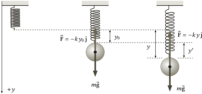
Figura 4.8: Objeto preso em uma mola pendurada.
