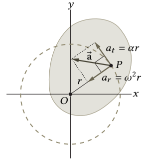
Figura 1.5: Quando um corpo rígido gira em torno de um eixo fixo através de O , o ponto P experimenta uma componente tangencial de aceleração linear a_t e uma componente radial de aceleração linear a_r .
