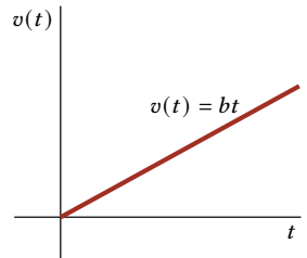
Figura 4.8: Gráfico da velocidade em função do tempo obtida no Exemplo 4.1 .
