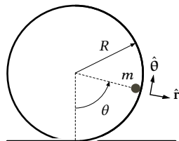
Figura 5.19: Partícula em um loop vertical.
