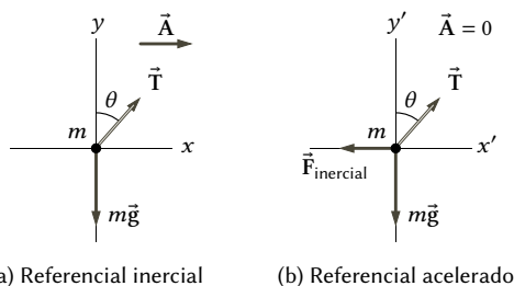
(a) Referencial inercial
