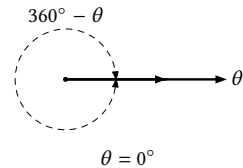
Figura 2.17: Ângulo entre vetores.
