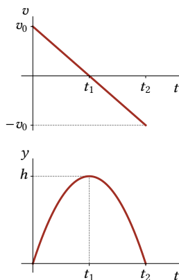
Figura 4.12: Gráficos da posição e velocidade para o movimento de um objeto que é lançado para cima em t = 0 com velocidade inicial v_0 , atinge a altura máxima h em t = t_1 e em seguida desce em queda livre até atingir a posição inicial em t = t_2 .
