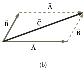
Figura 2.3: Duas regras geométricas para a adição de vetores. (a) Regra do polígono. (b) Regra do paralelogramo.
