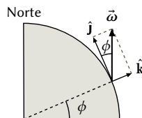
Figura 8.13: Sistema de coordenadas para o exemplo de queda livre.
