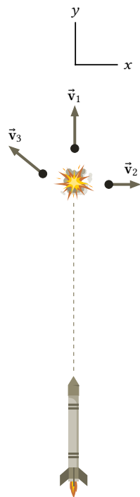
Figura 6.5: Foguete lançado verticalmente explode em três fragmentos de mesma massa.
