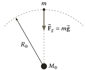
Figura 3.4: Força gravitacional sobre um corpo de massa m nas proximidades da superfície da Terra.
