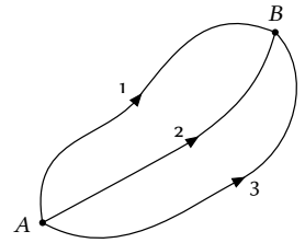
Figura 7.6: O trabalho realizado por uma força conservativa independe da trajetória.
