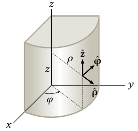
Figura 2.10: Vetores direcionais no sistema de coordenadas cilíndricas.
