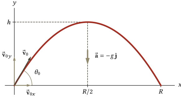
Figura 4.13: Se a resistência do ar for ignorada, a trajetória de um projétil é uma parábola.
