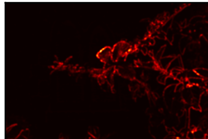
Saliency ( \mathcal{S} )
