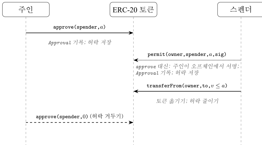
그림 2.1: ERC-20 허락의 한살이예요. approve 나 서명으로 대신하는 permit (점선), 해도 되고 안 해도 되는 transferFrom , 그리고 허락 거두기로 이어져요. 엔도스랭크 화살표 하나는 토큰마다 항목 하나씩 두고 이를 더한 값이에요. 각 항목은 관찰 기간 안에서 그 주인-스펜더 쌍의 가장 최근 Approval 이벤트에서 나와요. 이 항목은 AWP가 송금에 무게를 매기듯이, 그 허락의 나이(지난 시간)와 금액으로 무게를 매겨요. 나중 허락이 앞선 허락을 대신해요.
