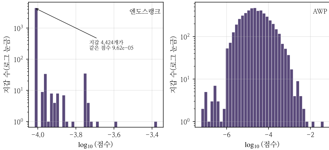
그림 4.2: 매칭 코호트( n = 5,521 )에서 엔도스랭크와 AWP 점수의 주변 분포예요. 점수가 0보다 큰 지갑을 \log_{10} 눈금으로 그렸고, 지갑 수도 로그 눈금이에요. 0점 지갑은 뺐어요. 이 지갑들에는 그 그래프의 화살표가 하나도 닿지 않아요. 엔도스랭크는 966개, AWP는 381개예요. 엔도스랭크에서는 4,424개 지갑이 허락을 받지 않은 지갑의 점수 9.62 \times 10^{-5} 를 함께 가지고, 그보다 위에 있는 것은 131개뿐이에요.
