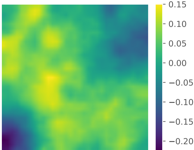
True u
