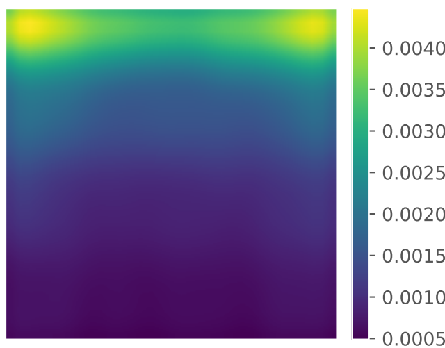
SI Var
