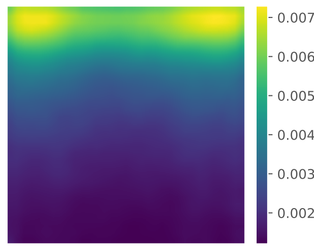
h-MALA Var
