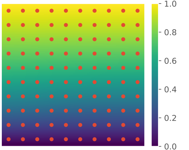
True State
