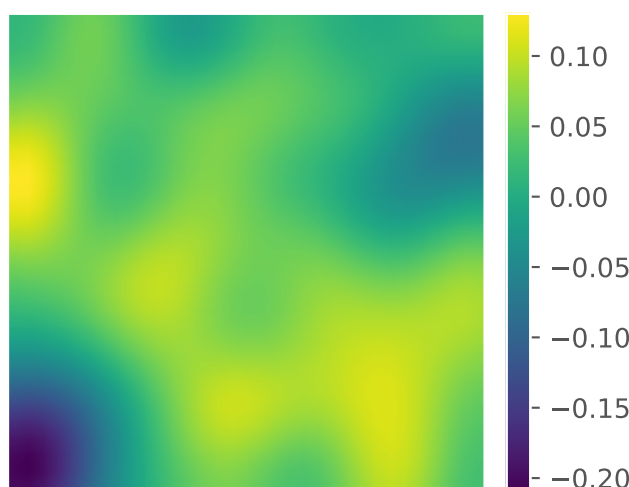
SI Mean
