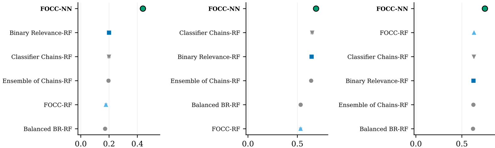
Reuters-21578 ( L=90 , general)
