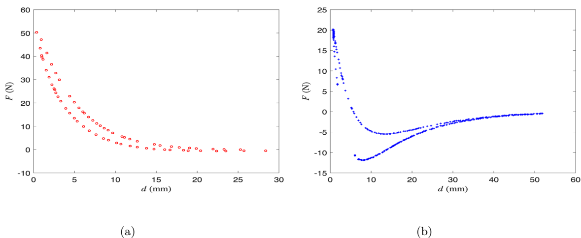
图 5: (a) 零场冷条件下磁悬浮力随距离的变化 (b) 场冷条件下磁悬浮力随距离的变化
