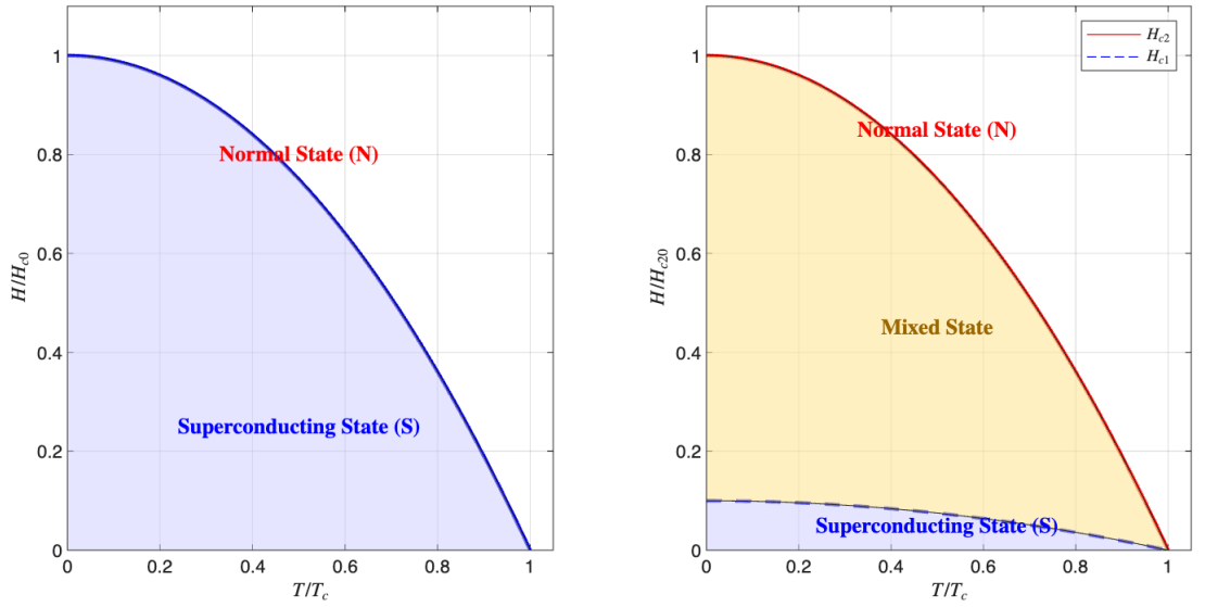
图 2: 两类超导体的 H - T 示意图 (左: 第一类; 右: 第二类)
