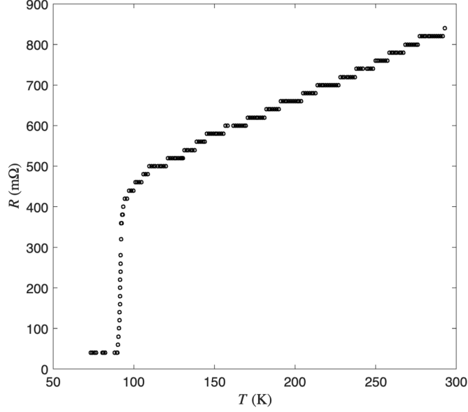
图 3: 实验测得的 R - T 超导转变曲线
