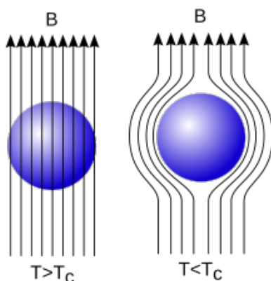
图 1: 迈斯纳效应示意图
