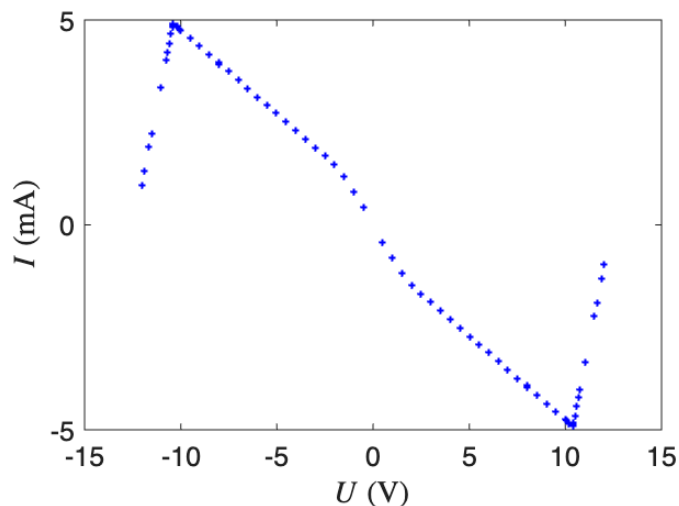
图 3: 非线性负阻实验数据散点图
