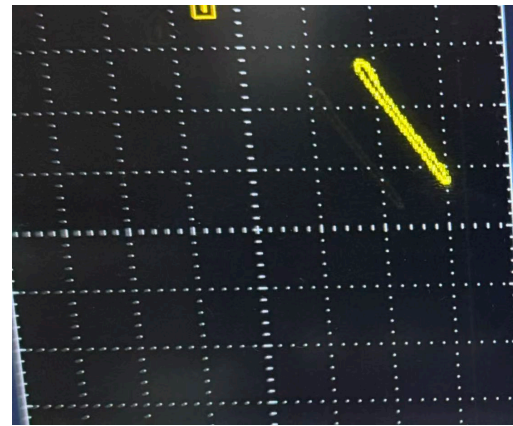
(b) 准同步实验图
