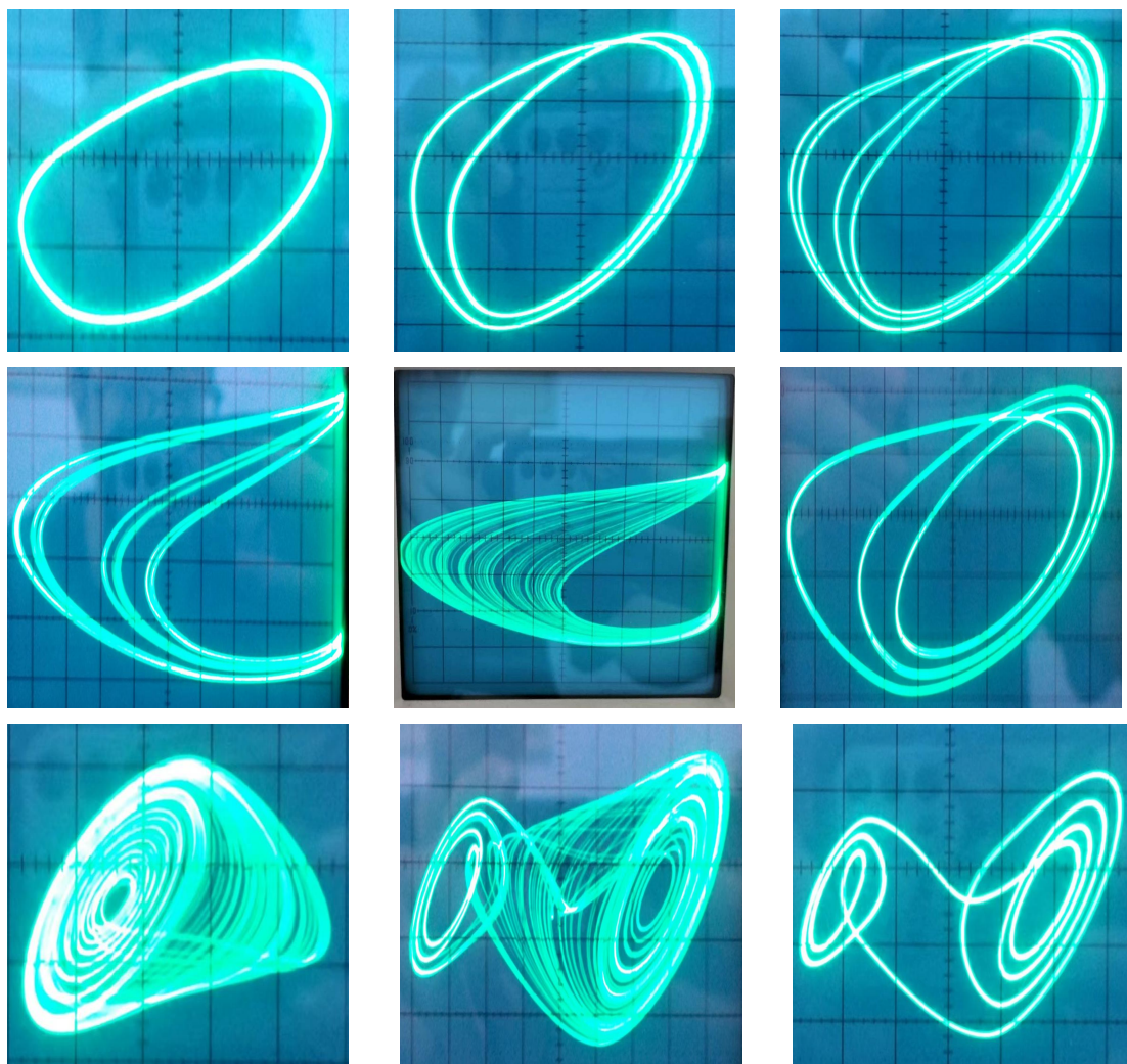
图 5: 电路状态的变化
