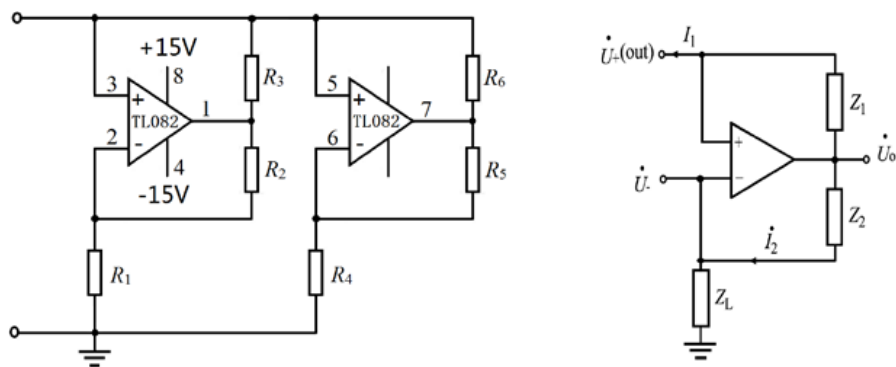
图 2: 非线性负阻示意图
