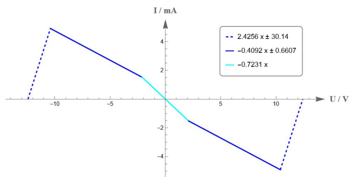
图 4: 非线性负阻实验数据拟合图
