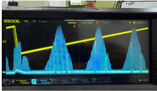
(a) 出光带宽的示波器示例
