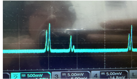
(b) 纵模分裂的双峰结构示例
