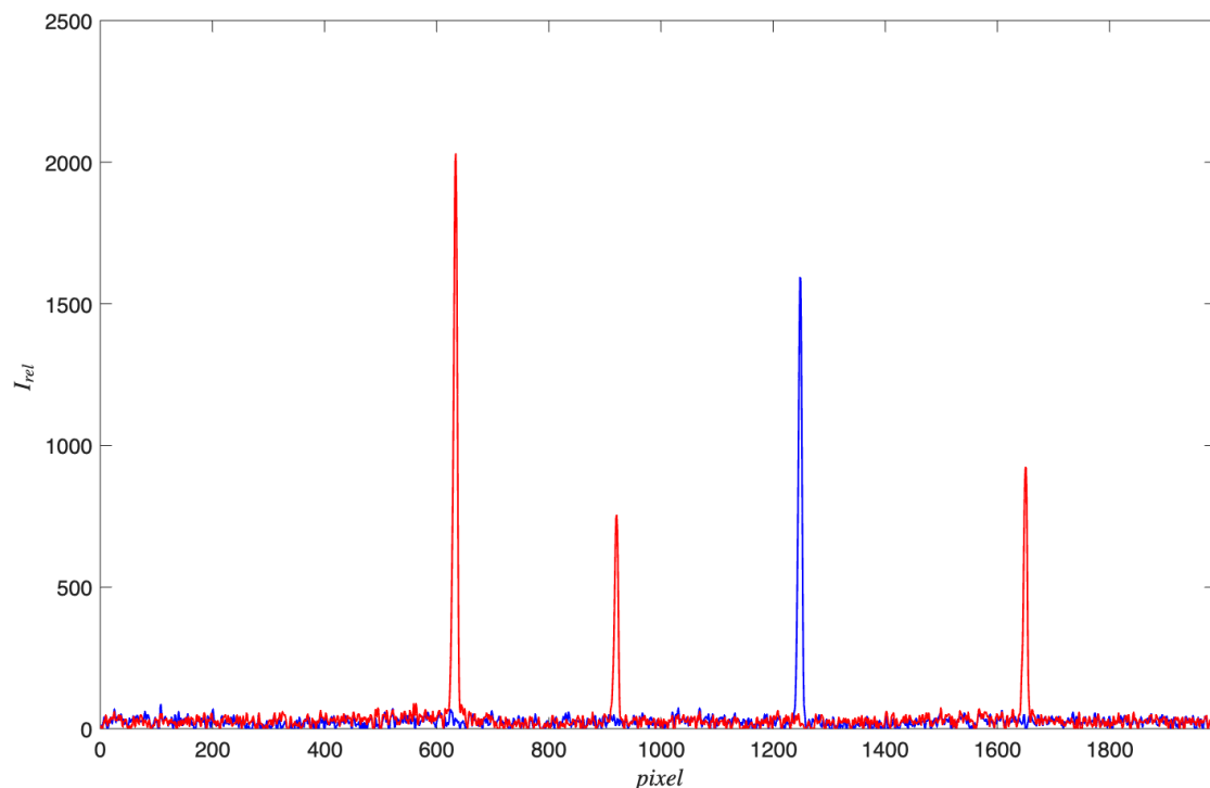
图 2: 使用 CCD 测得的 H_\alpha 谱线
