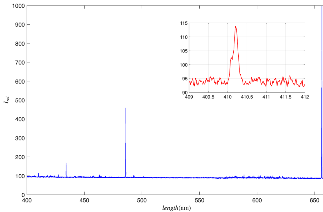
图 4: 使用 PMT 测得的氢氫谱线
