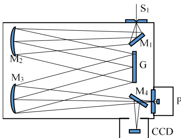
图 1: 光学多色仪示意图
