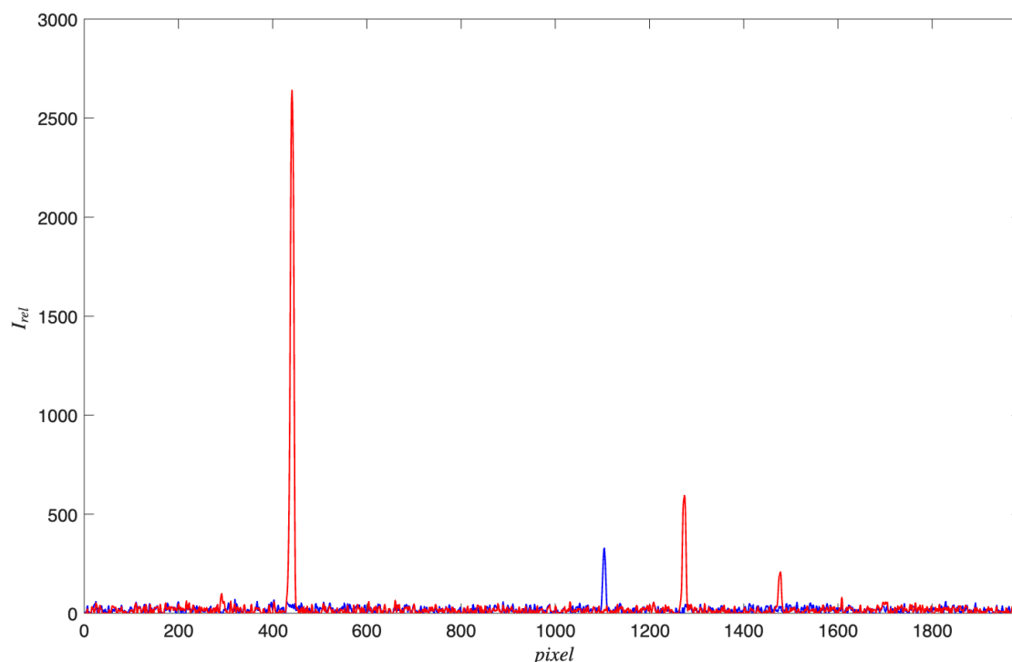
图 3: 使用 CCD 测得的 H_\delta 谱线
