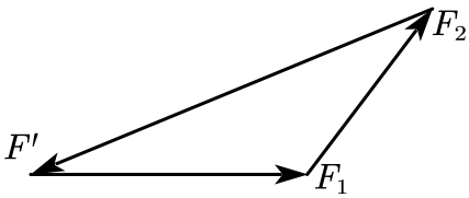
图 3.4: 力的三角形
