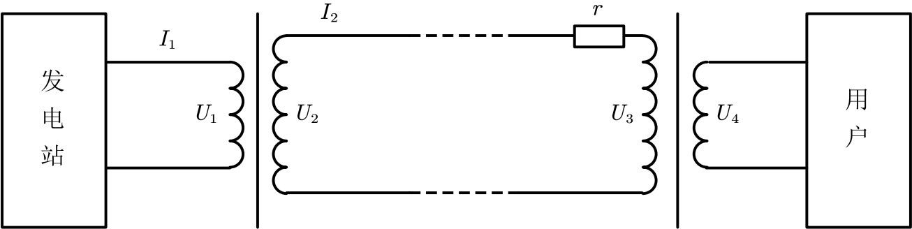
图 15.5: 高压输电示意图
