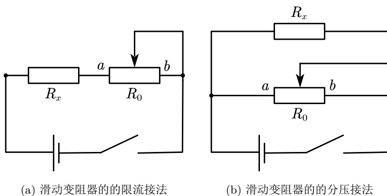
图 12.10: 滑动变阻器的限流接法和分压接法
