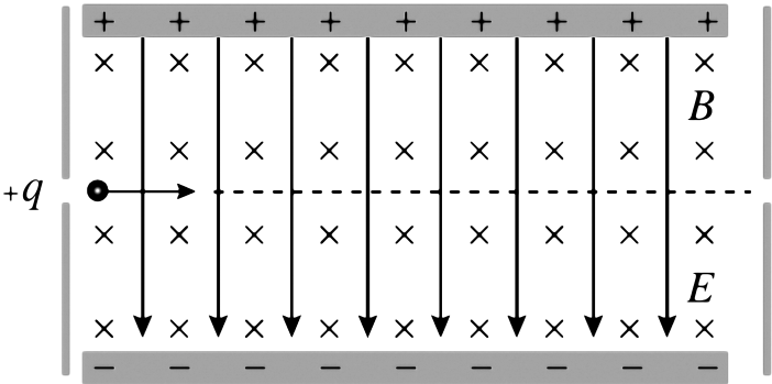
图 13.2: 速度选择器
