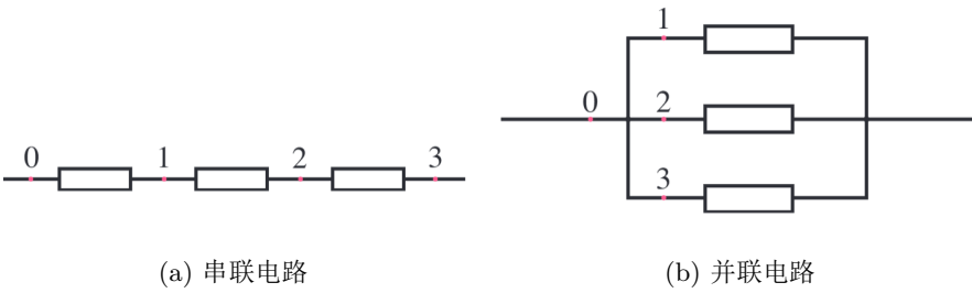
图 12.3: 串联和并联
