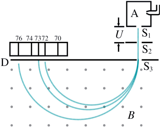
图 13.3: 质谱仪
