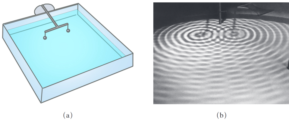
图 22.6: 水波实验发生器与水波干涉图样
