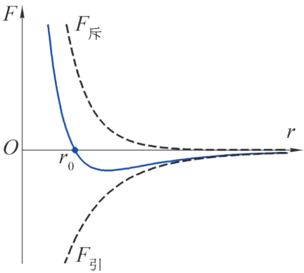
图 18.1: 分子间作用力
