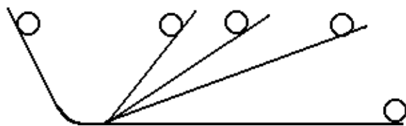
图 4.1: 伽利略的理想实验
