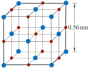
图 19.3: 氯化钠晶体的微观结构
