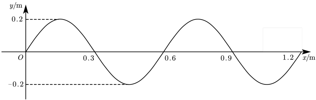
图 22.3: 横波的图像
