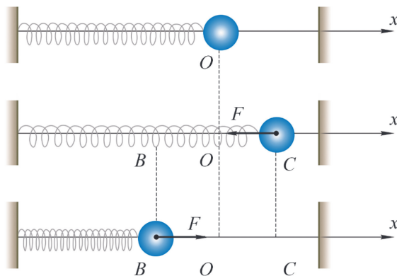
图 21.3: 弹簧振子的受力分析
