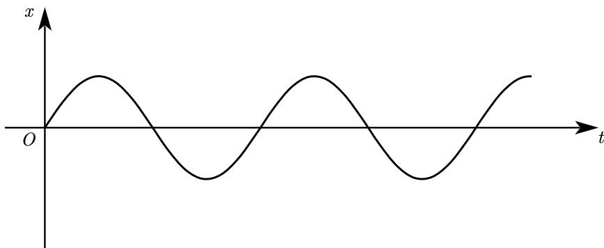
图 21.2: 振动图像
