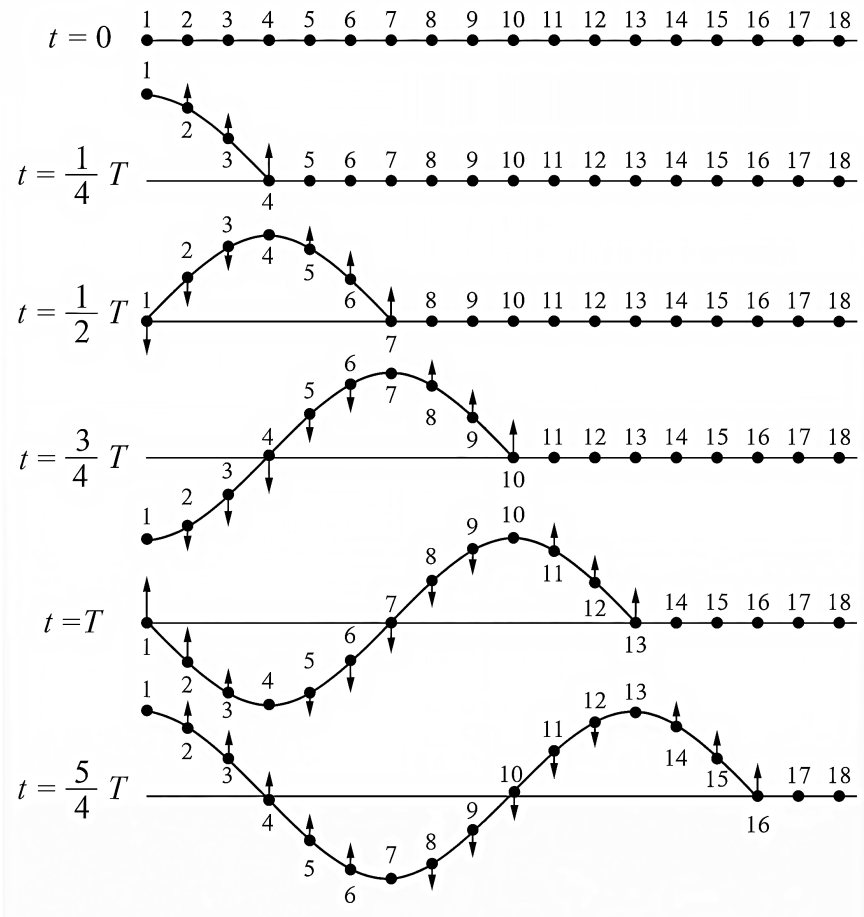
图 22.2: 绳波在不同时刻的波形
