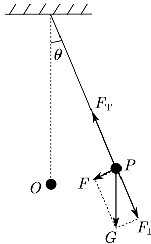
图 21.5: 分析单摆的回复力
