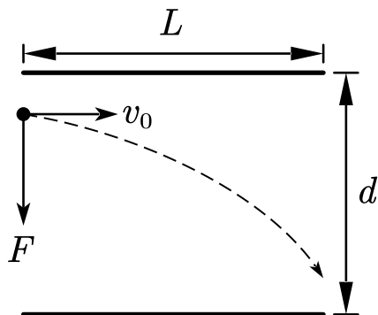
图 11.7: 匀强电场中的类平抛运动
