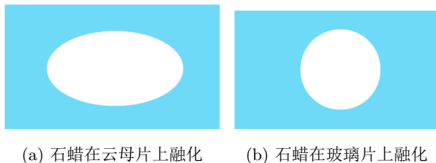
图 19.2: 石蜡在云母片和玻璃片上的熔化情况
