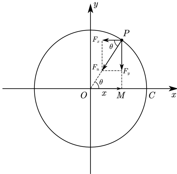
图 21.4: 简谐运动与圆周运动的关系
