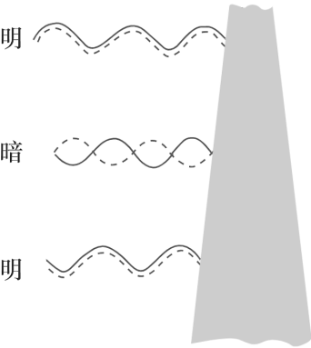
图 23.5: 肥皂液膜的反射光
