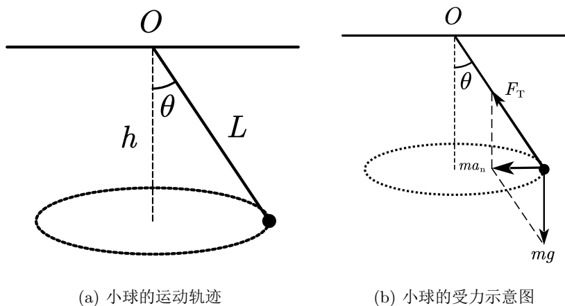
图 7.1: 圆锥摆模型
