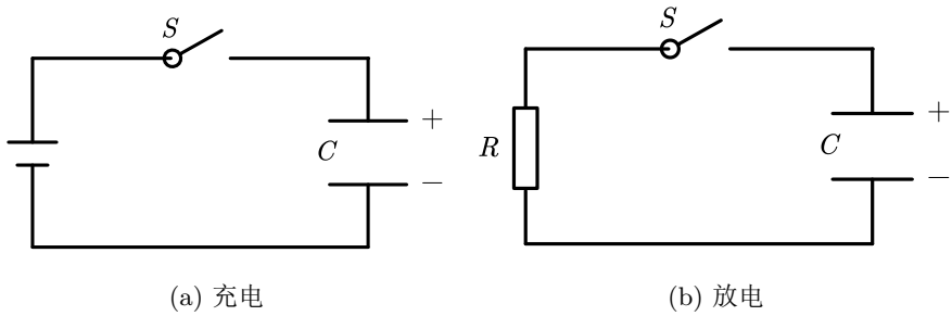
图 11.4: 平行板电容器的充放电
