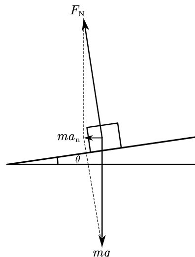
图 7.3: 火车的轨道
