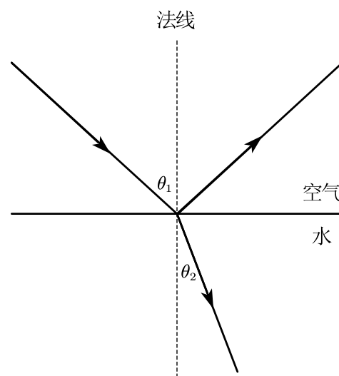
图 23.1: 光的反射和折射
