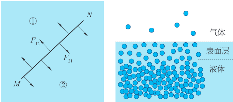
图 19.4: 液体的表面张力
