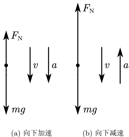
图 4.2: 下蹲的加速阶段和减速阶段
