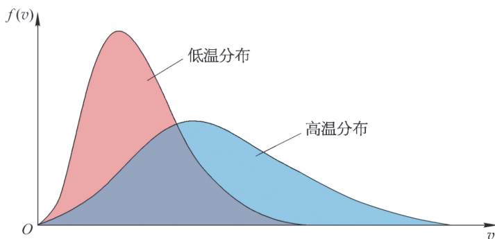
图 18.2: 气体分子速率分布曲线
