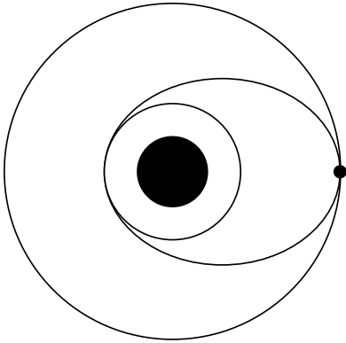
图 8.2: 卫星的变轨问题
