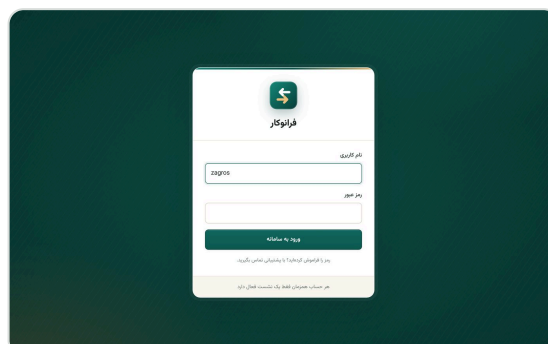
صفحه‌ی ورود
