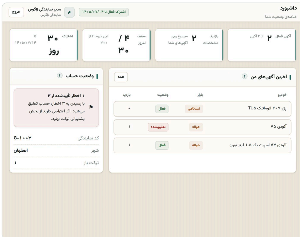
داشبورد نمایندگی
