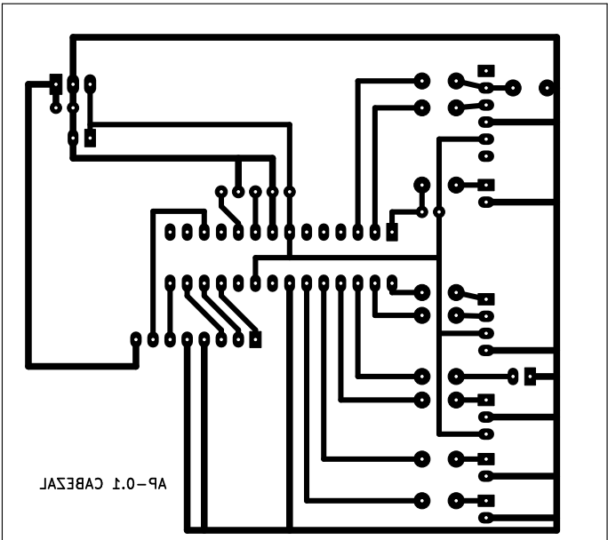
Cabezal 2
