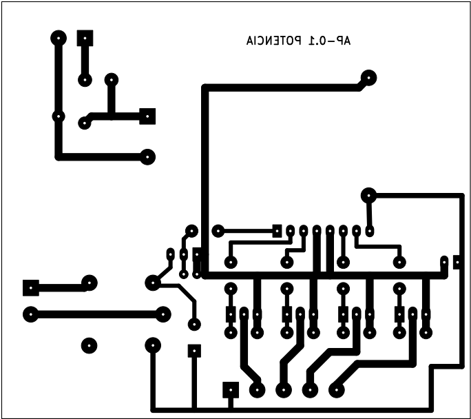
Potencia 2
