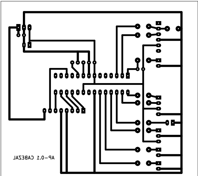
Cabezal 1
