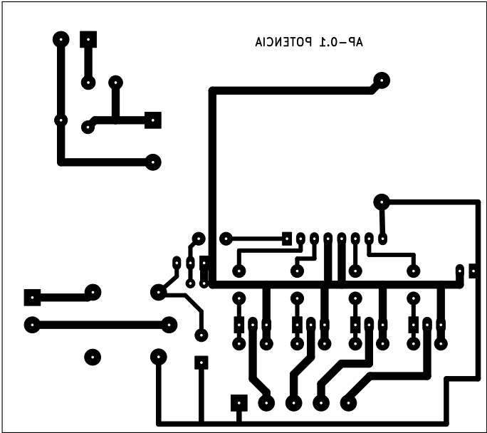
Potencia 1
