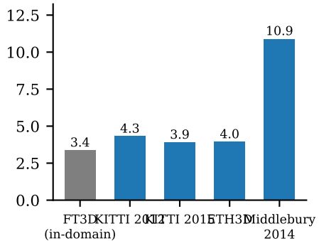
D1-all (%)
