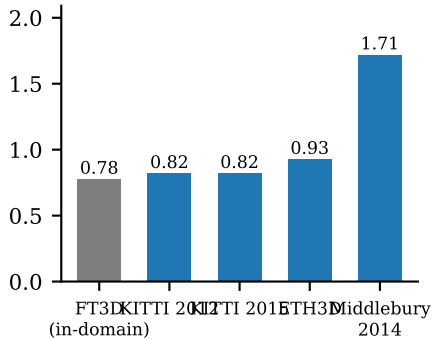
EPE (px)
