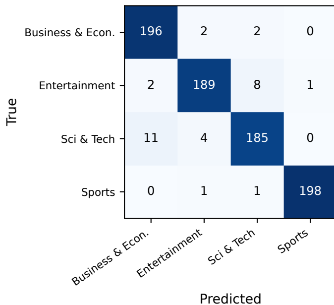
Gemma-2-2B (acc 0.960)
