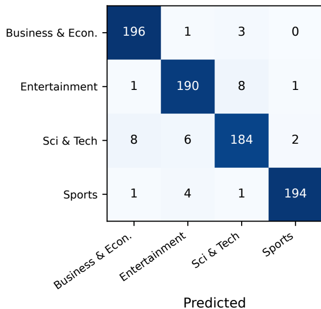
Llama-3.2-3B (acc 0.955)
