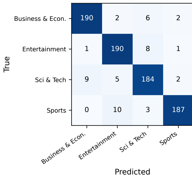
Qwen2.5-3B (acc 0.939)
