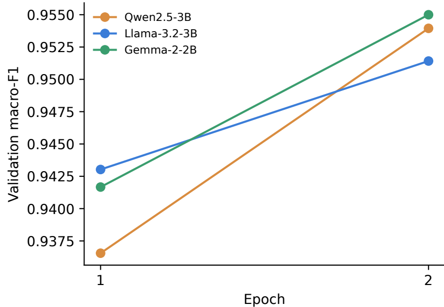
Validation macro-F1 per epoch
