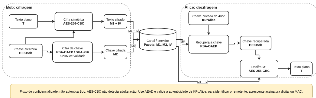
Figura 7: Proteção híbrida da mensagem: AES cifra os dados e RSA-OAEP protege a chave de dados
