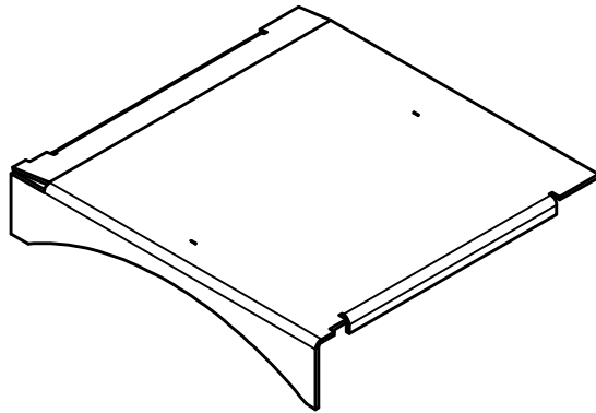
ISO SCALE 1/16
