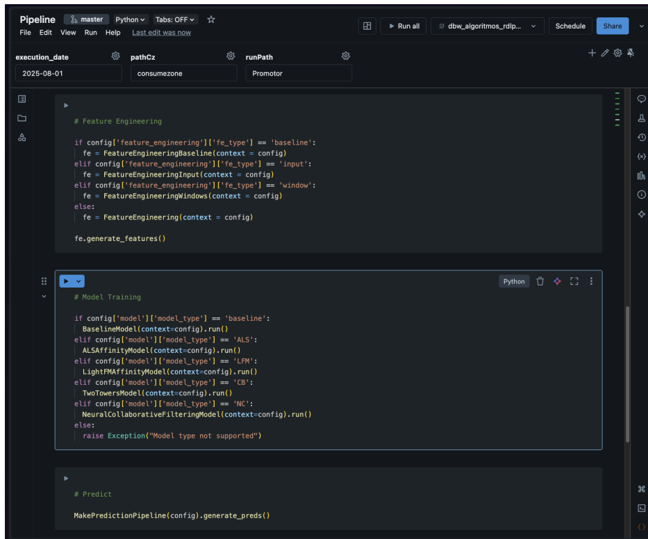
FIGURA 3.12. Pipeline de ejecución.
