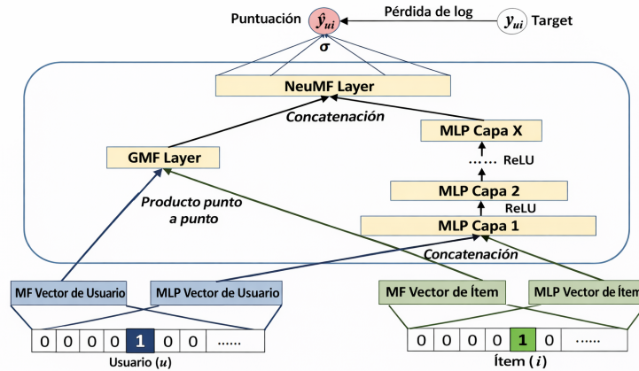
FIGURA 3.11. Arquitectura del modelo Neural Collaborative Filtering híbrido 2 .
