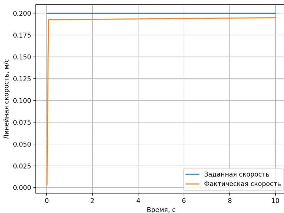
Рисунок 8 — Заданные и фактические значения линейной скорости при прямолинейном движении
