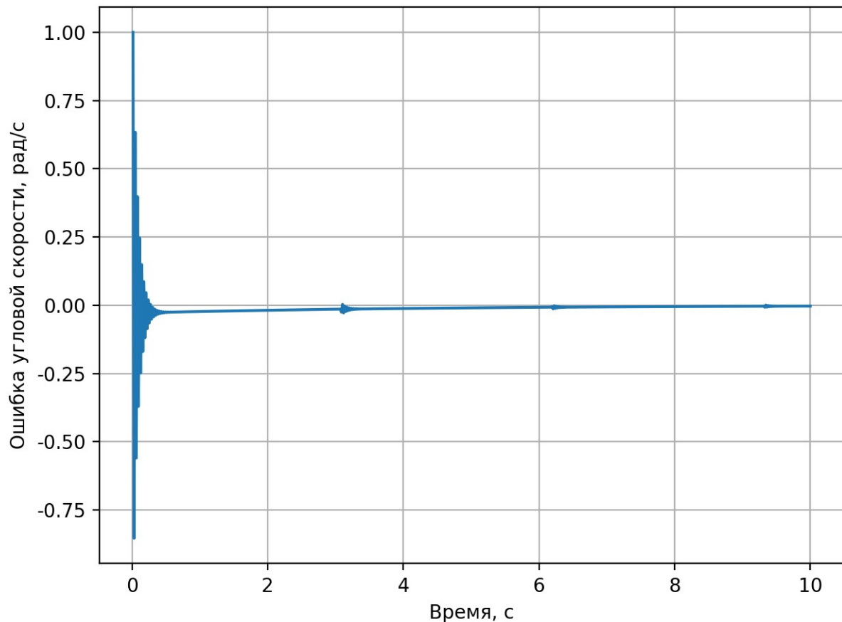
Рисунок 11 — Отклонение угловой скорости от заданного значения при повороте на месте
