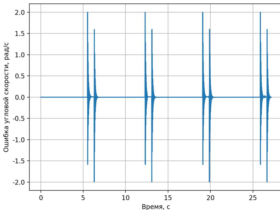
Рисунок 17 — Отклонение угловой скорости от заданного значения при движении по квадратной траектории
