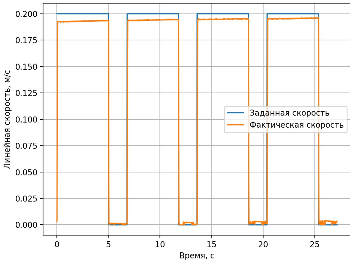
Рисунок 22 — Заданная и измеренная линейная скорость при аппаратно-программной проверке
