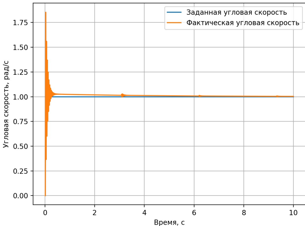
Рисунок 10 — Заданные и фактические значения угловой скорости при повороте на месте
