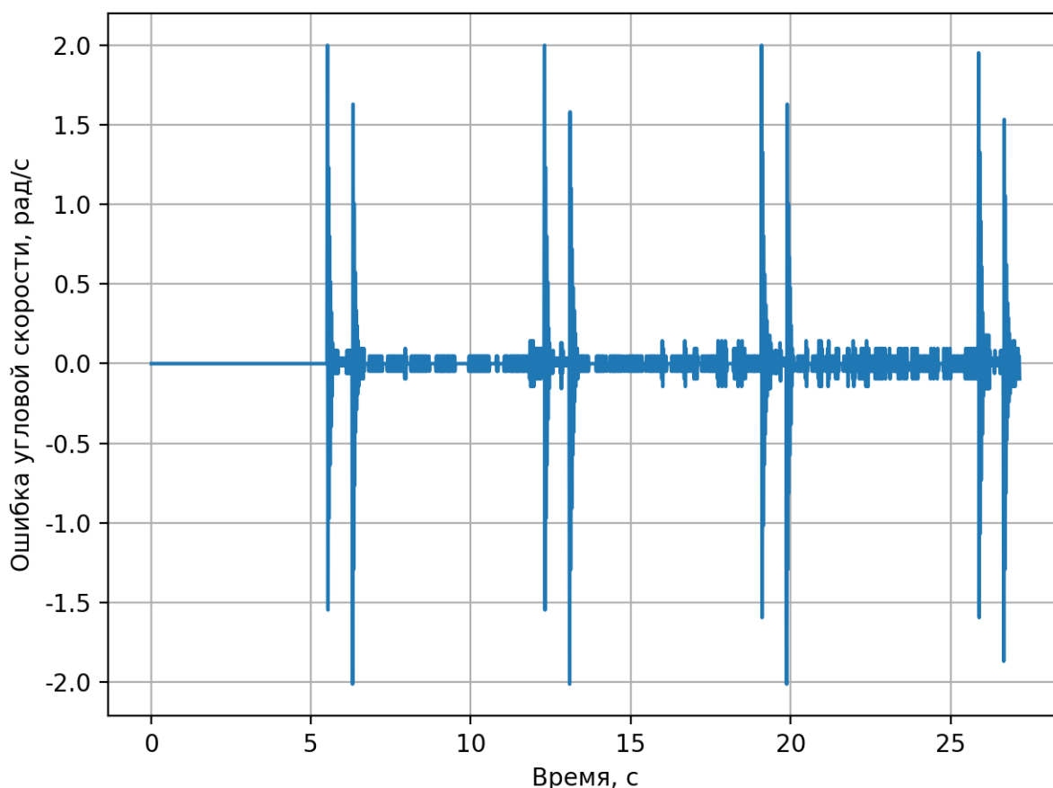
Рисунок 25 — Ошибка регулирования угловой скорости при аппаратно-программной проверке
