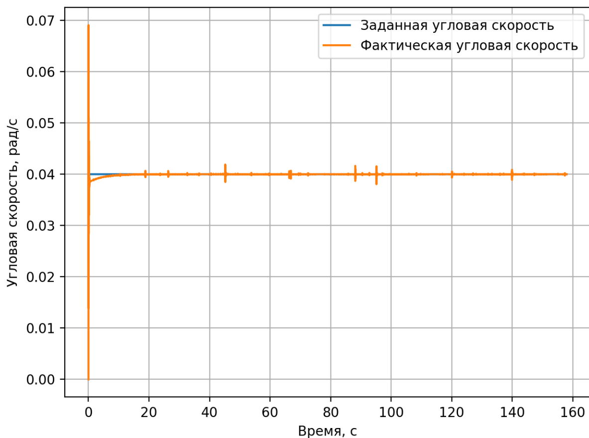
Рисунок 14 — Заданные и фактические значения угловой скорости при движении по окружности
