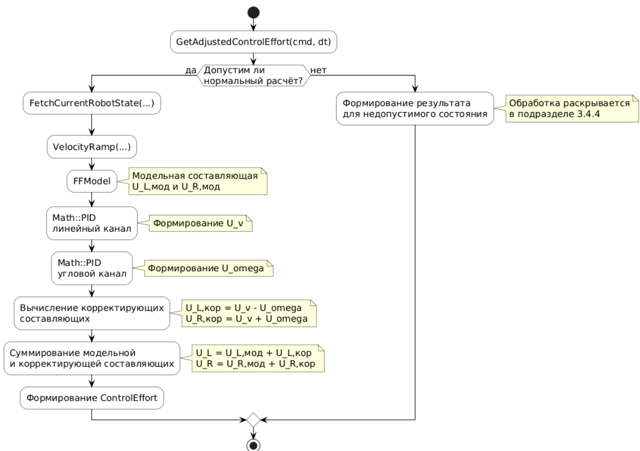
Рисунок 5 — Блок-схема вычисления управляющего воздействия
