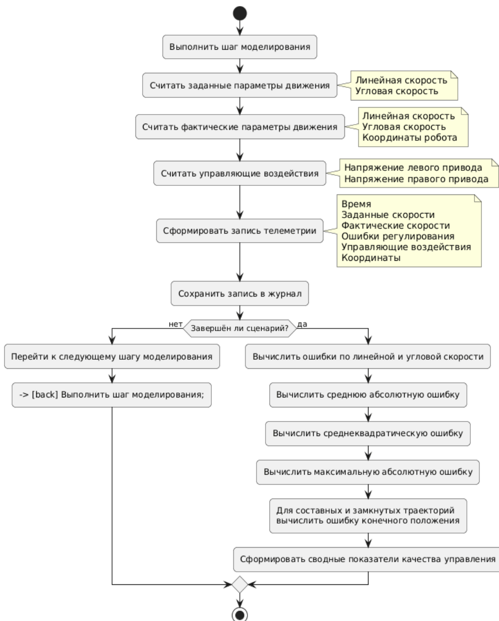
Рисунок 7 — Структура формирования телеметрии и расчёта показателей качества
