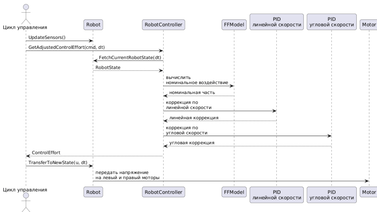
Рисунок 3 — Последовательность выполнения одного шага управления
