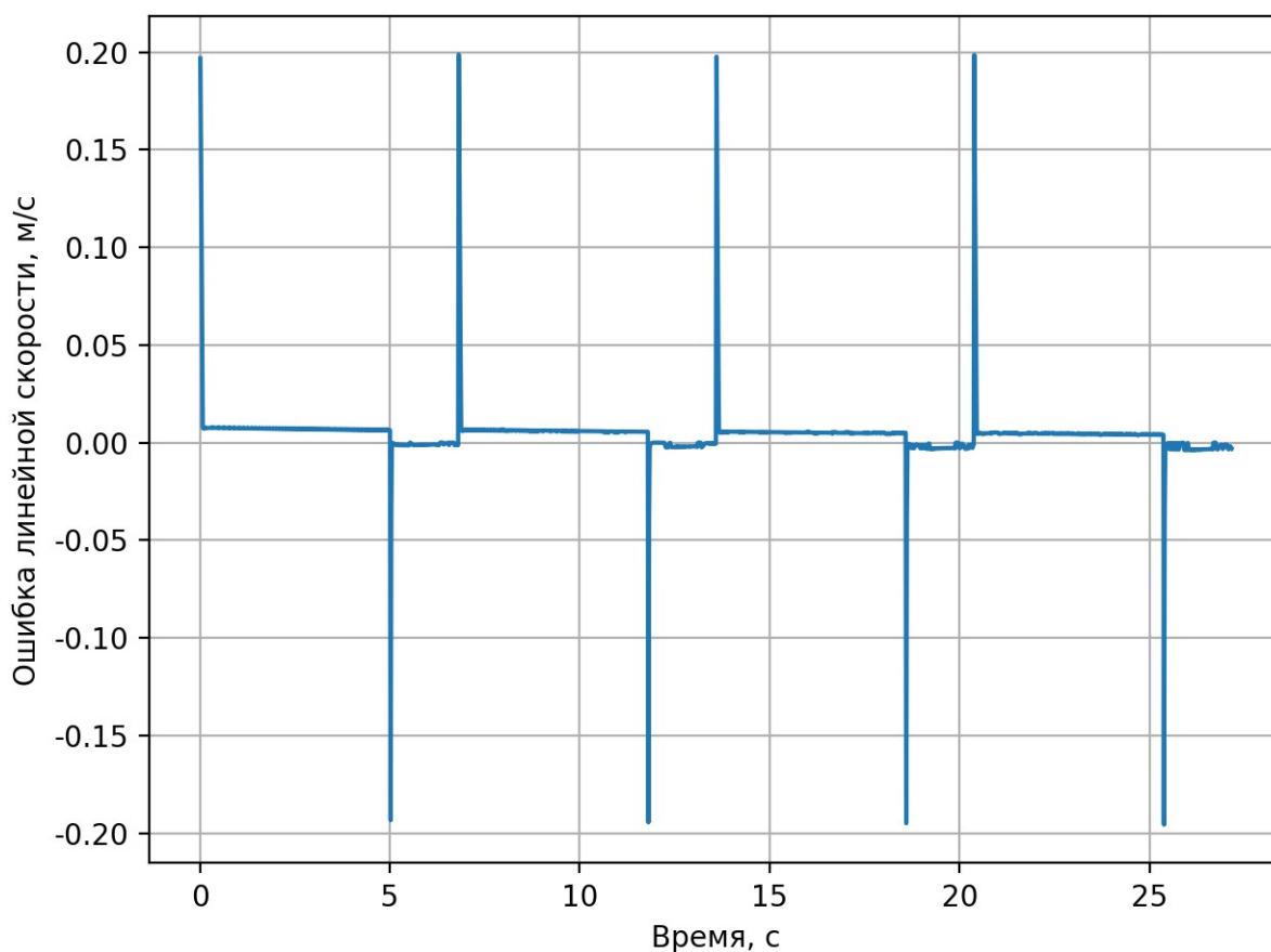
Рисунок 24 — Ошибка регулирования линейной скорости при аппаратно-программной проверке
