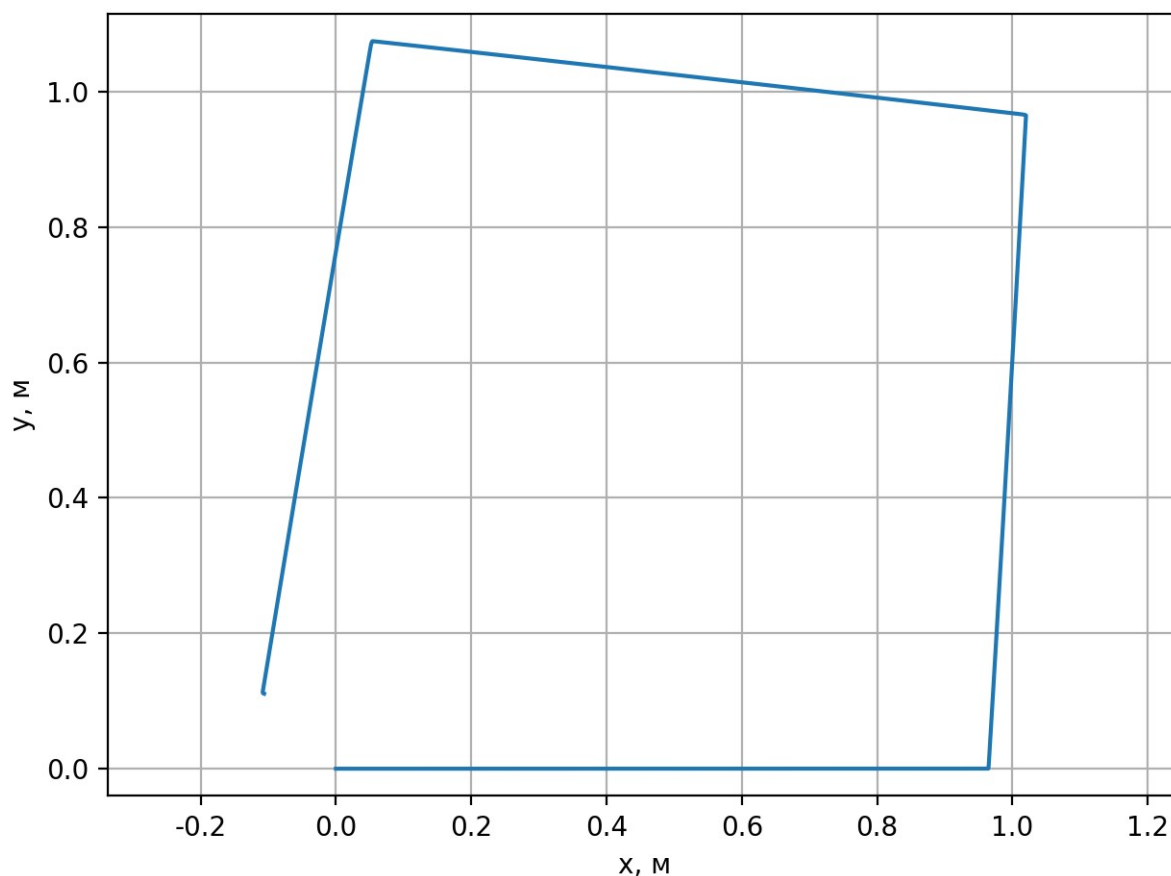
Рисунок 21 — Траектория движения мобильной платформы при аппаратно-программной проверке
