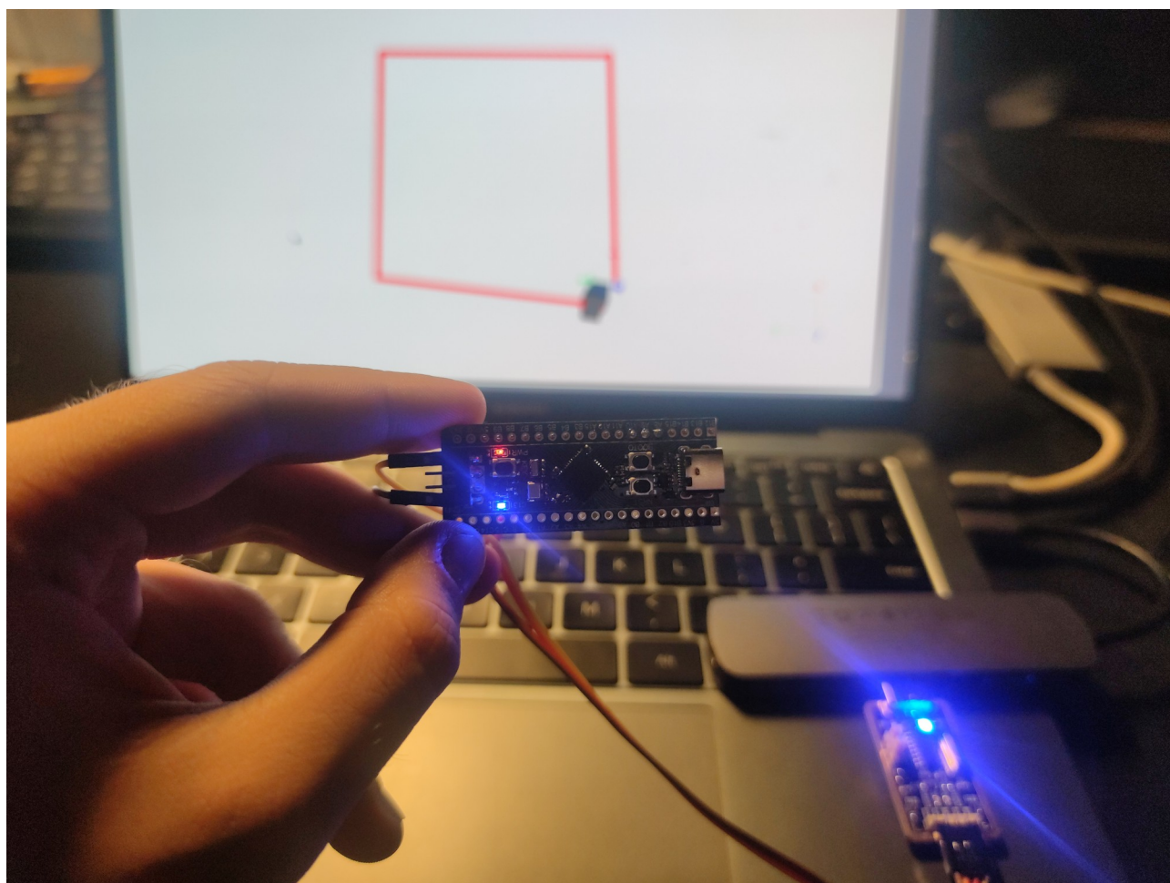
Рисунок 18 — Общий вид аппаратно-программного стенда для проверки программы управления
