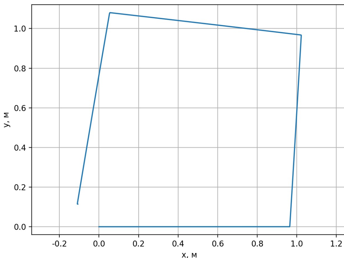
Рисунок 15 — Траектория движения мобильной платформы при движении по квадратной траектории
