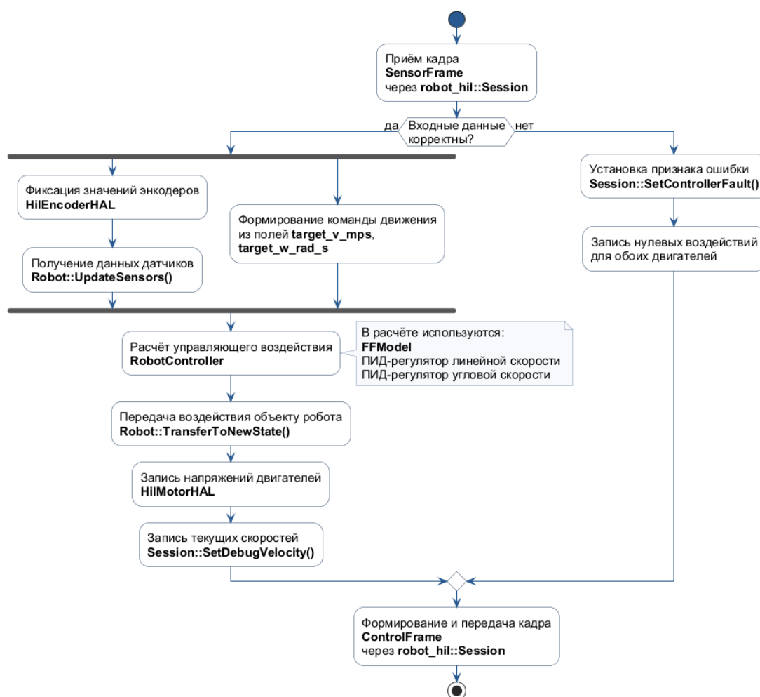
Рисунок 20 — Выполнение управляющего шага в прошивке STM32
