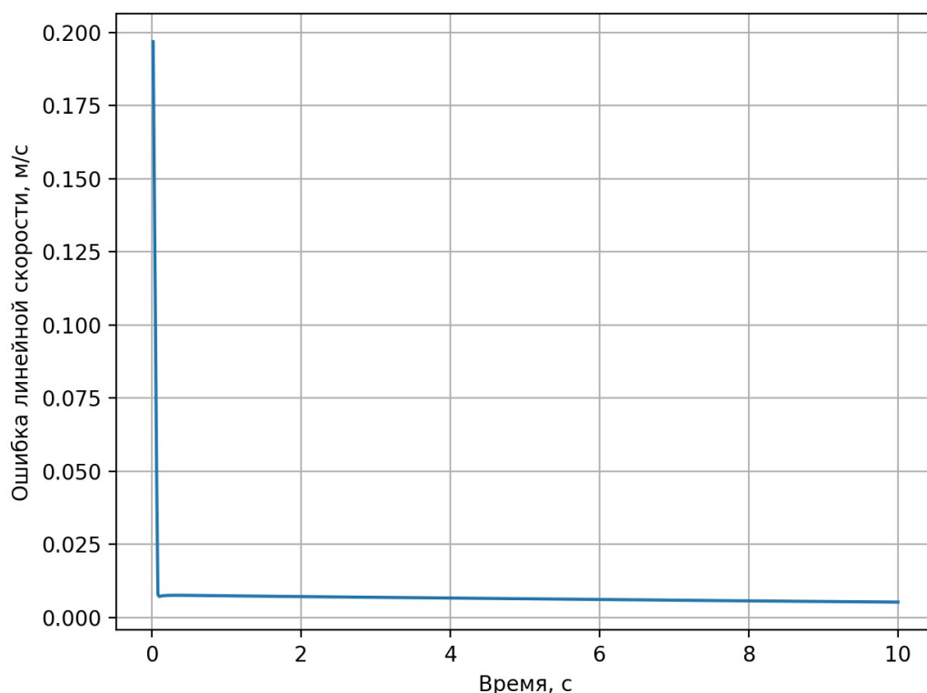
Рисунок 9 — Отклонение линейной скорости от заданного значения при прямолинейном движении
