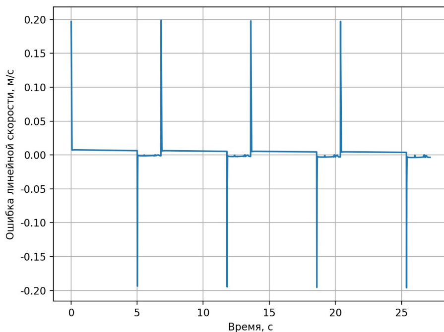
Рисунок 16 — Отклонение линейной скорости от заданного значения при движении по квадратной траектории
