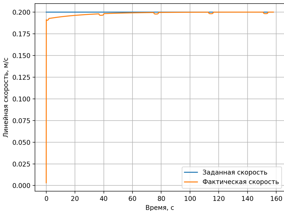
Рисунок 13 — Заданные и фактические значения линейной скорости при движении по окружности
