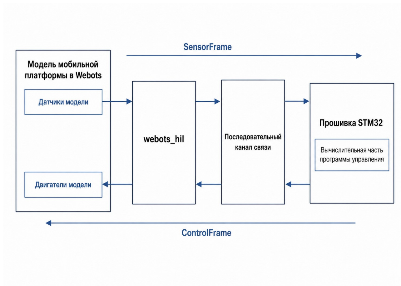
Рисунок 23 — Структура аппаратно-программного контура проверки
