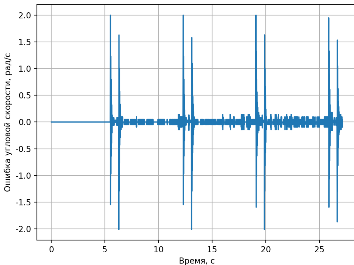
Рисунок 29 — Ошибка регулирования угловой скорости при аппаратно-программной проверке
