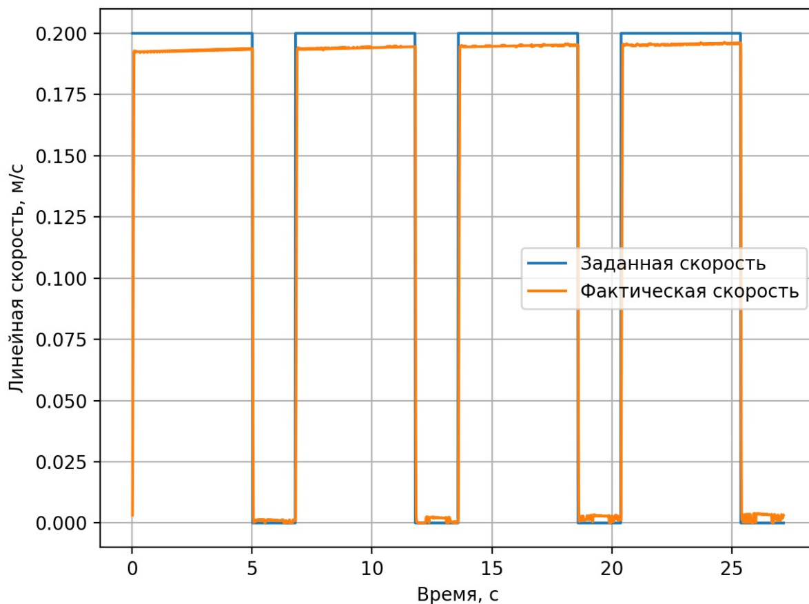
Рисунок 26 — Заданная и измеренная линейная скорость при аппаратно-программной проверке
