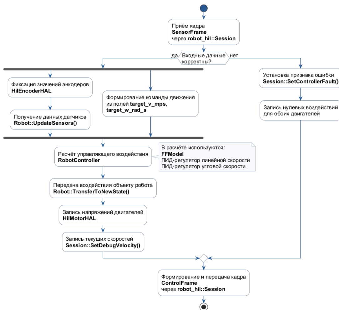
Рисунок 24 — Выполнение управляющего шага в прошивке STM32
