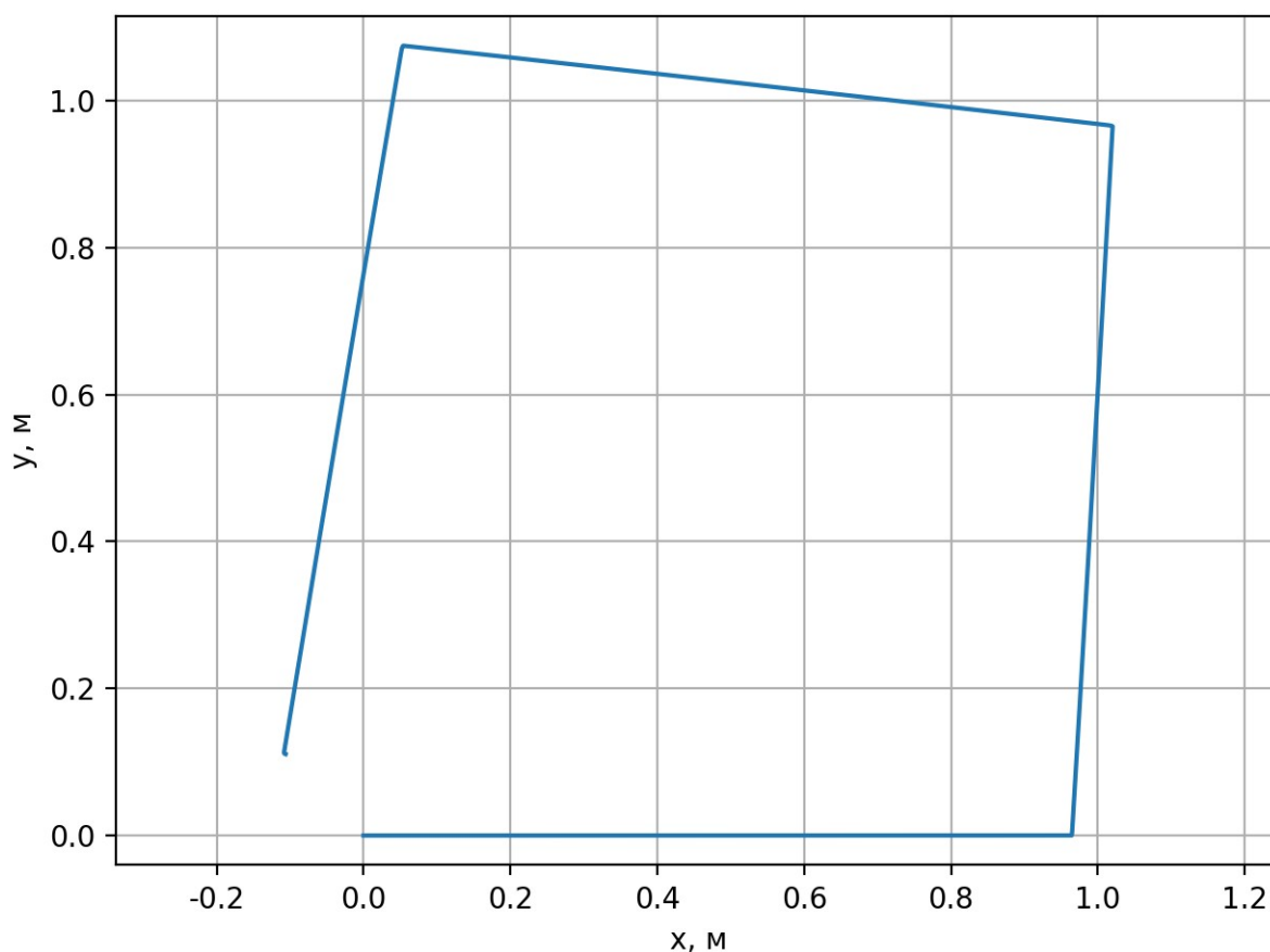
Рисунок 25 — Траектория движения мобильной платформы при аппаратно-программной проверке
