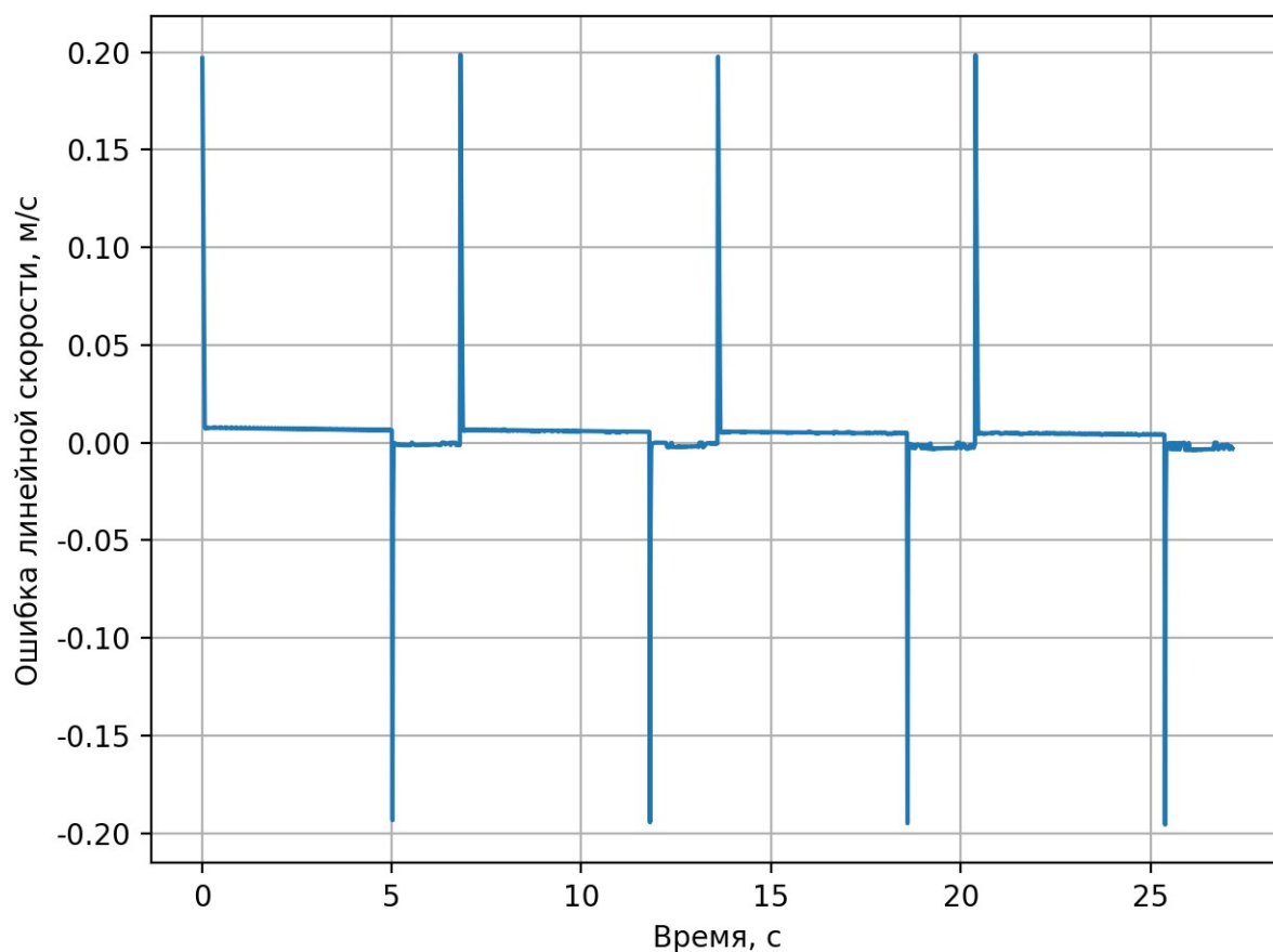
Рисунок 28 — Ошибка регулирования линейной скорости при аппаратно-программной проверке
