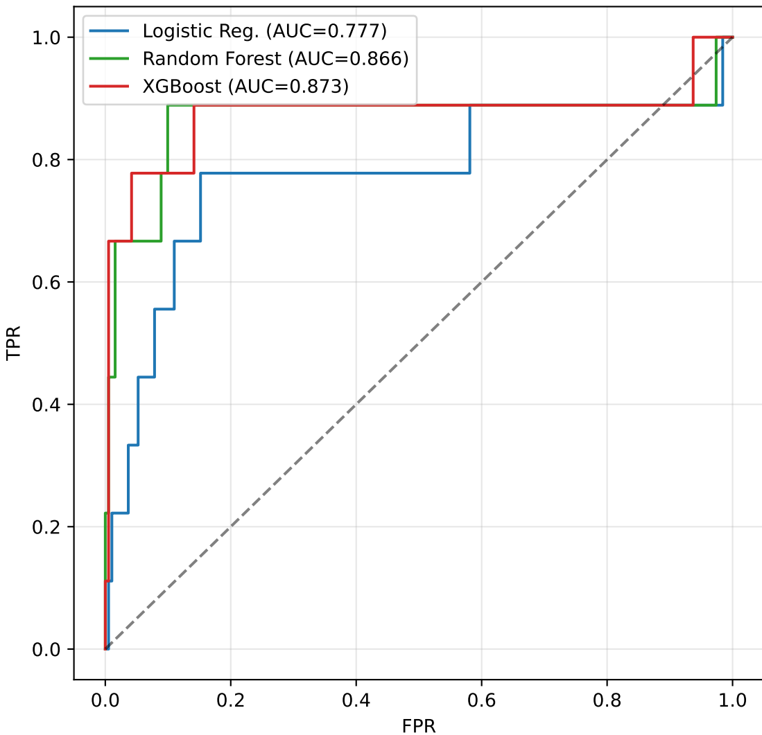
ROC — test
