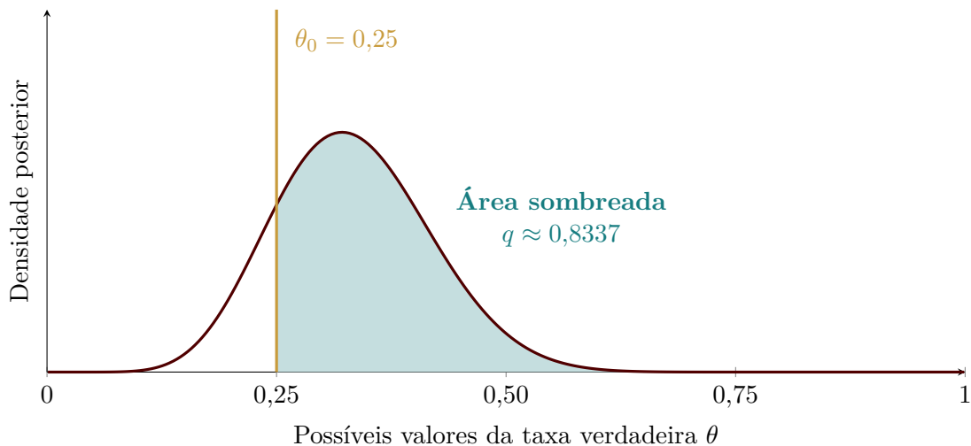
Figure 1: Distribuição posterior \text{Beta}(10, 20) . A região sombreada representa P(\theta > 0,25 \mid D) .
