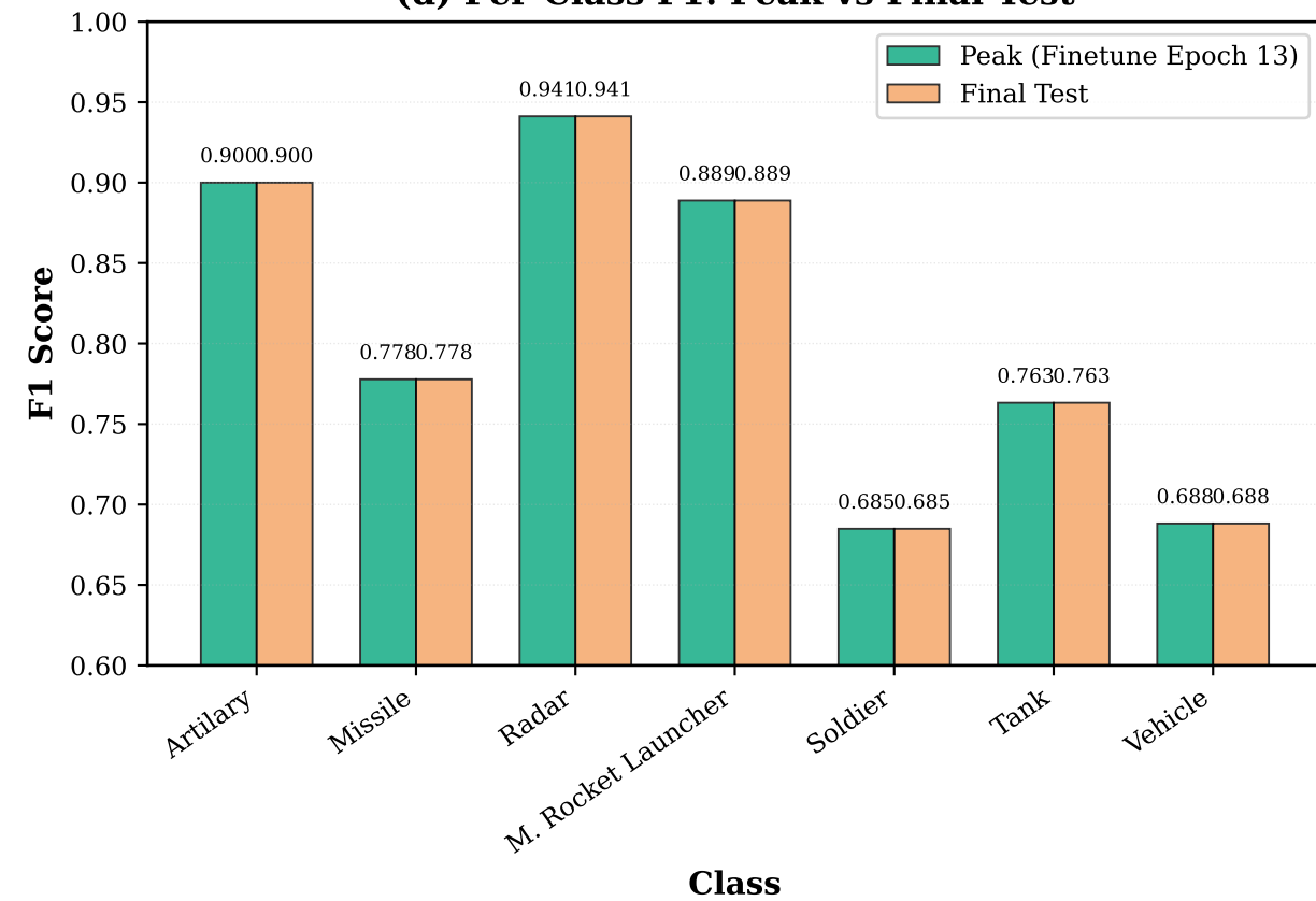
(d) Per-Class F1: Peak vs Final Test
