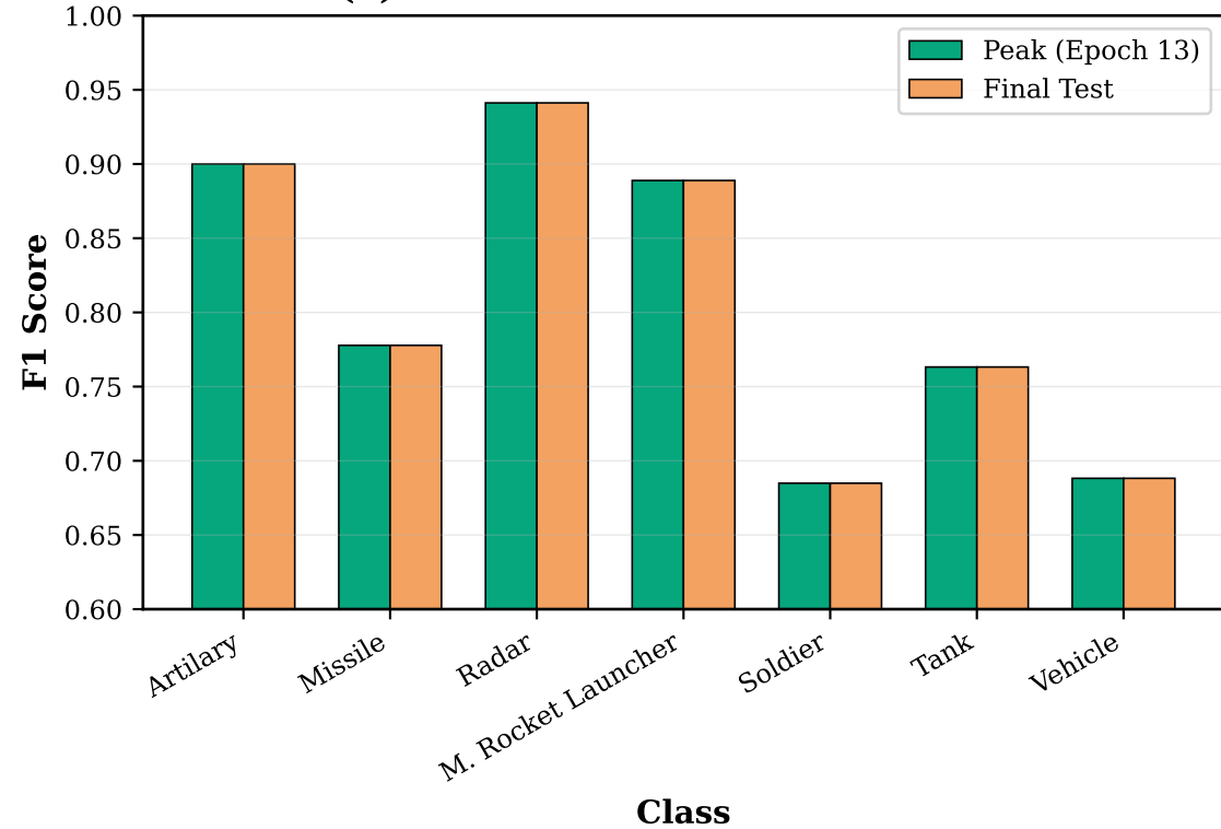
(d) Per-Class F1: Peak vs Final Test
