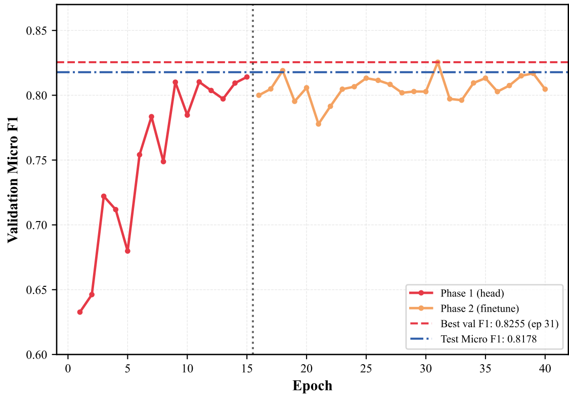
(b) Validation F1 Over Training
