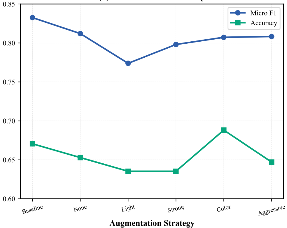
(a) Micro F1 and Accuracy
