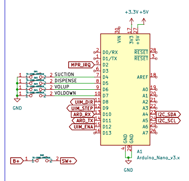
Arduino_Nano_v3.x
