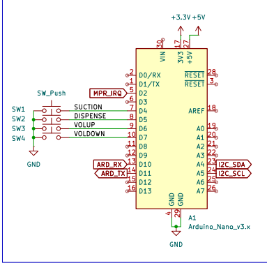
Arduino_Nano_v3.x
