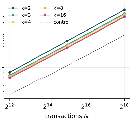
BLAKE2s-256
