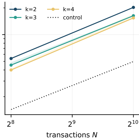
BLAKE2s-256
