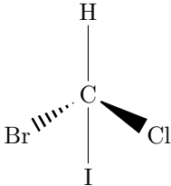
bromocloroyodometanc
