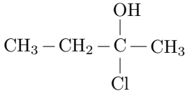
2-clorobutan-2-ol
