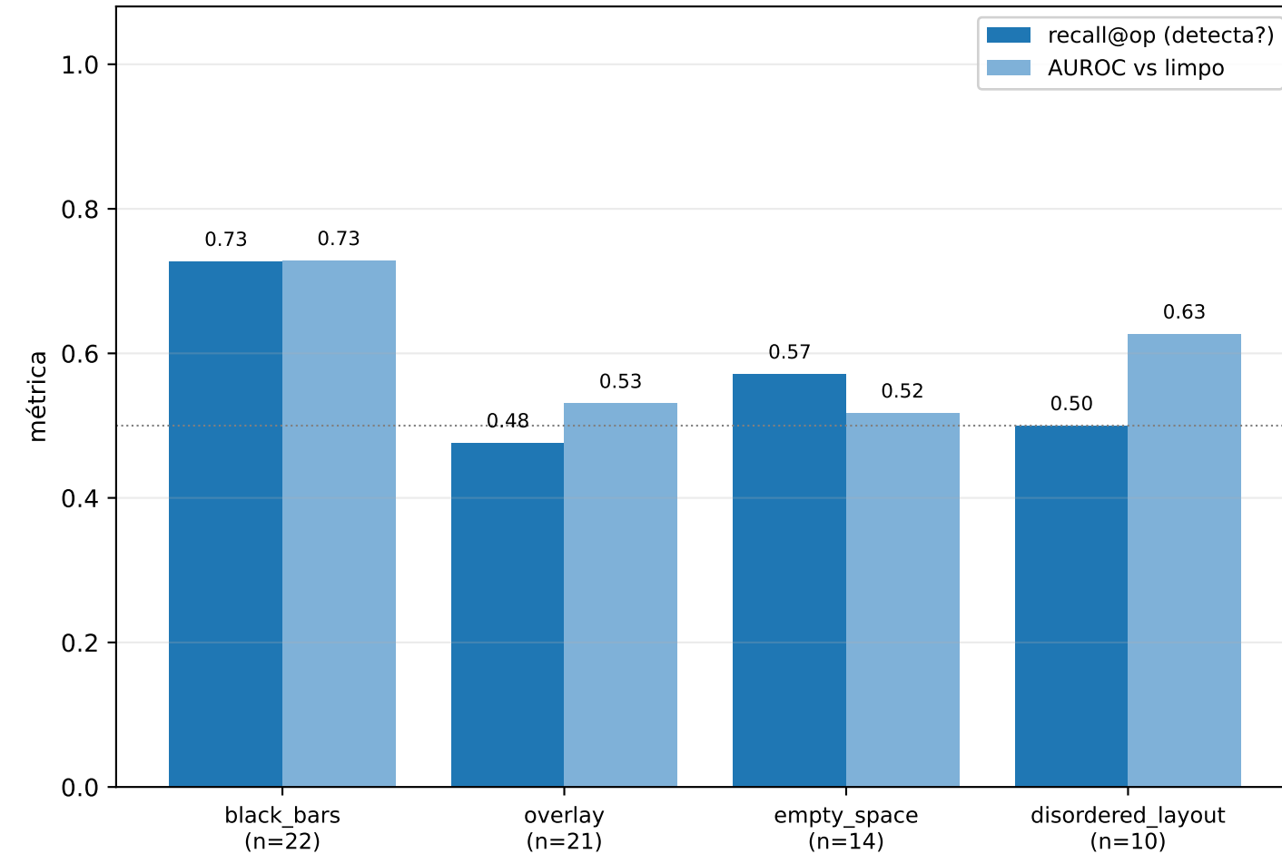
Estágio 1 — DETECÇÃO por classe (o gate pega o erro?)
