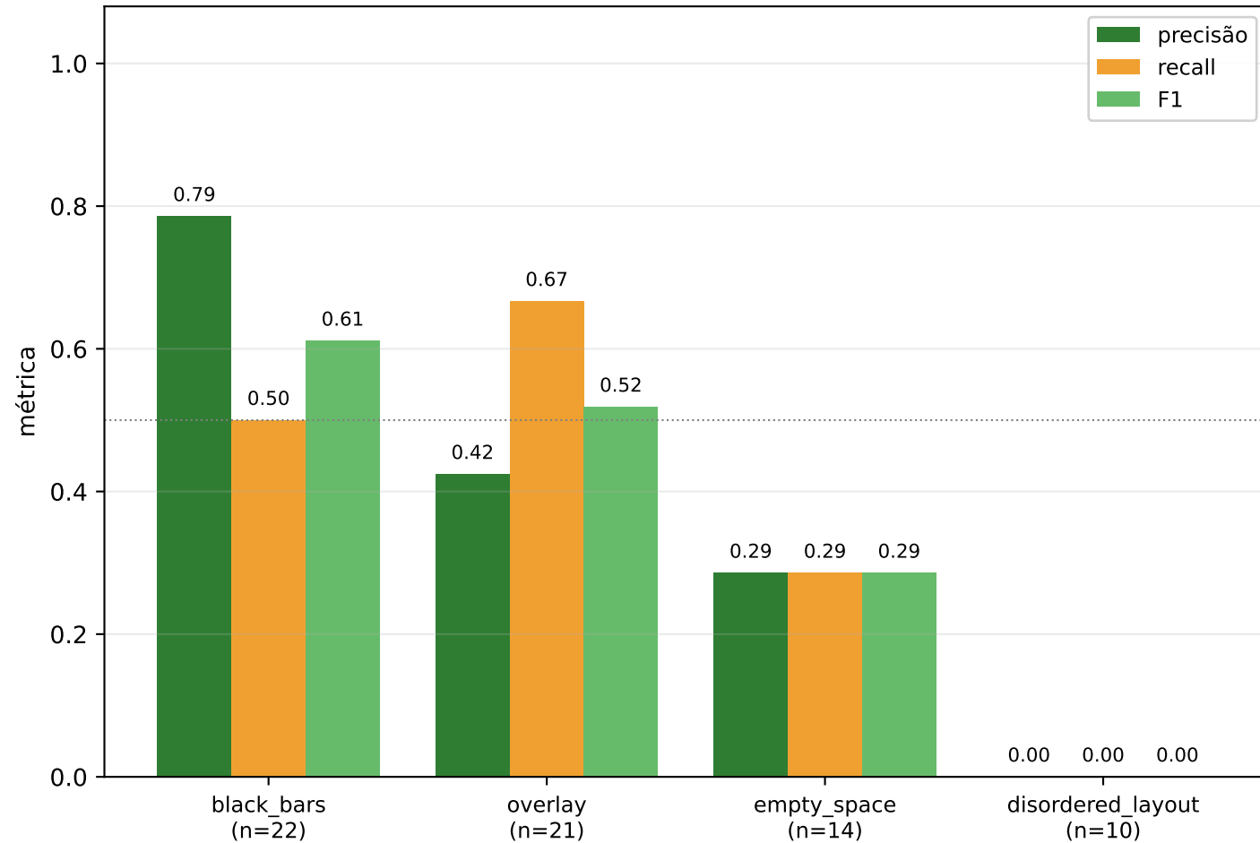
Estágio 2 — CLASSIFICAÇÃO por classe (acerta a categoria?)
