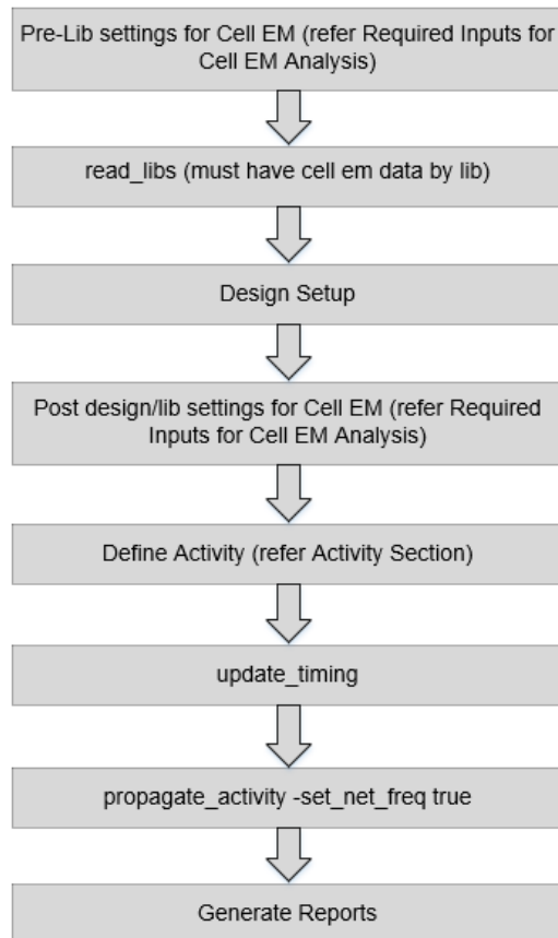
Figure 4-120 Cell EM STA Flow
