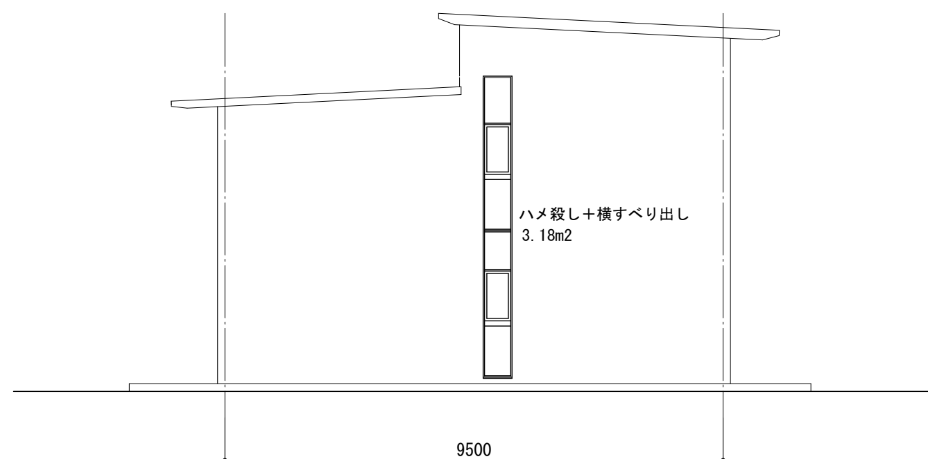
西立面图 1:100
