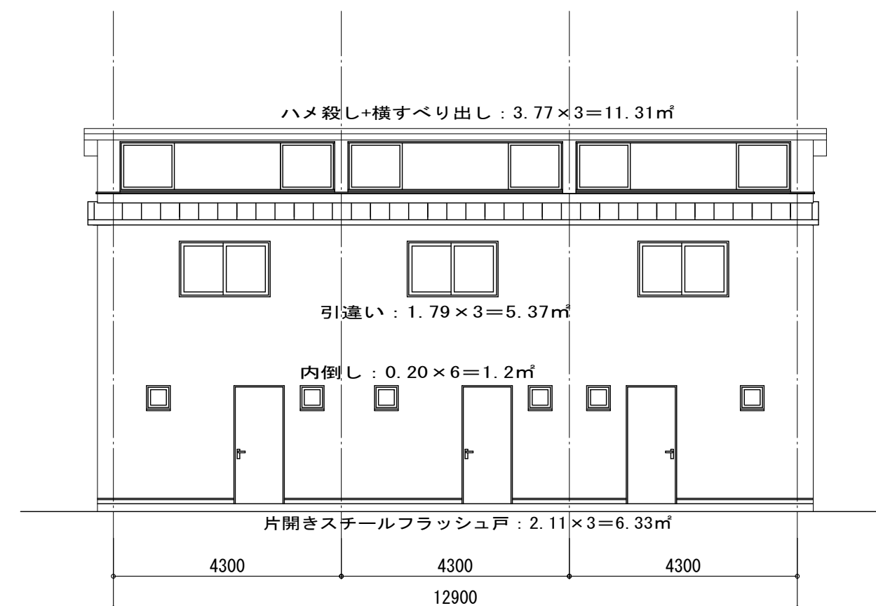
北立面图 1:100
