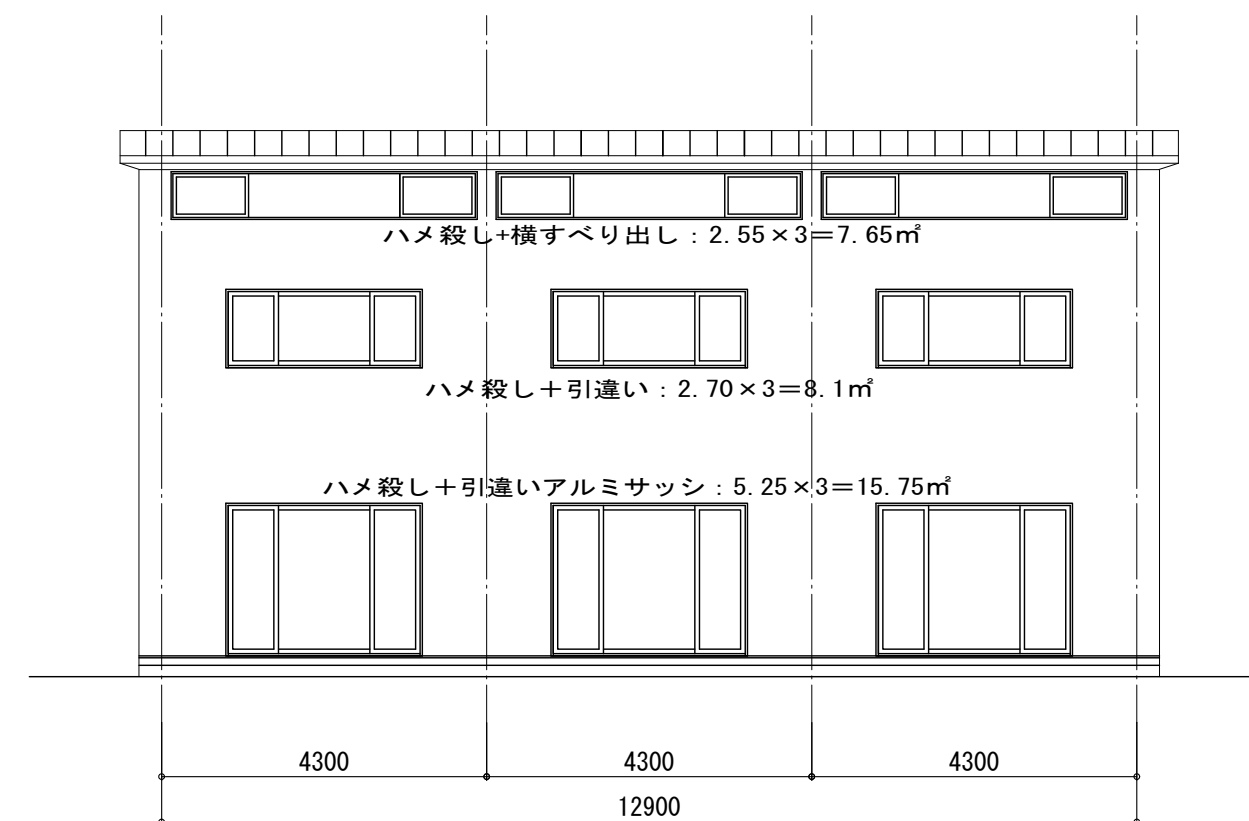
南立面图 1:100
