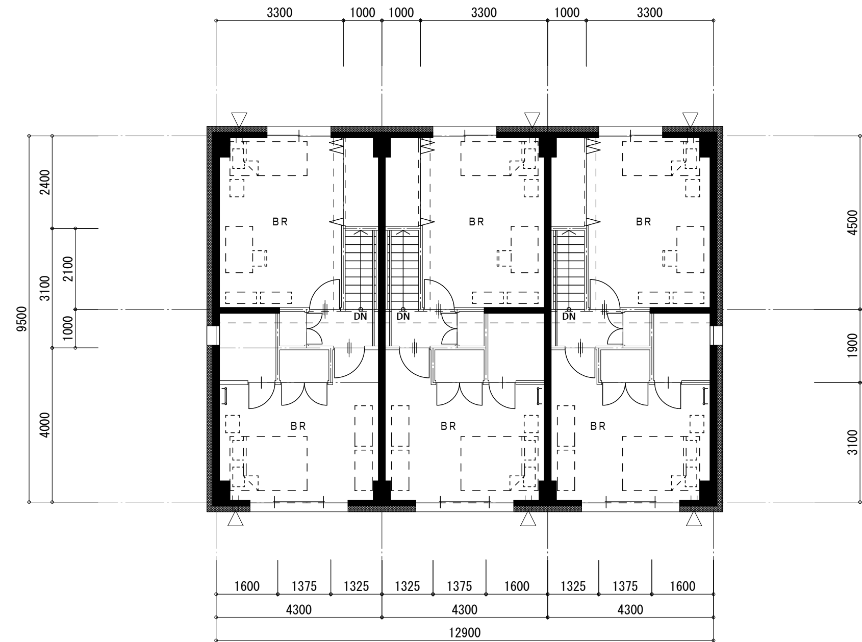
2階平面図 1:100
