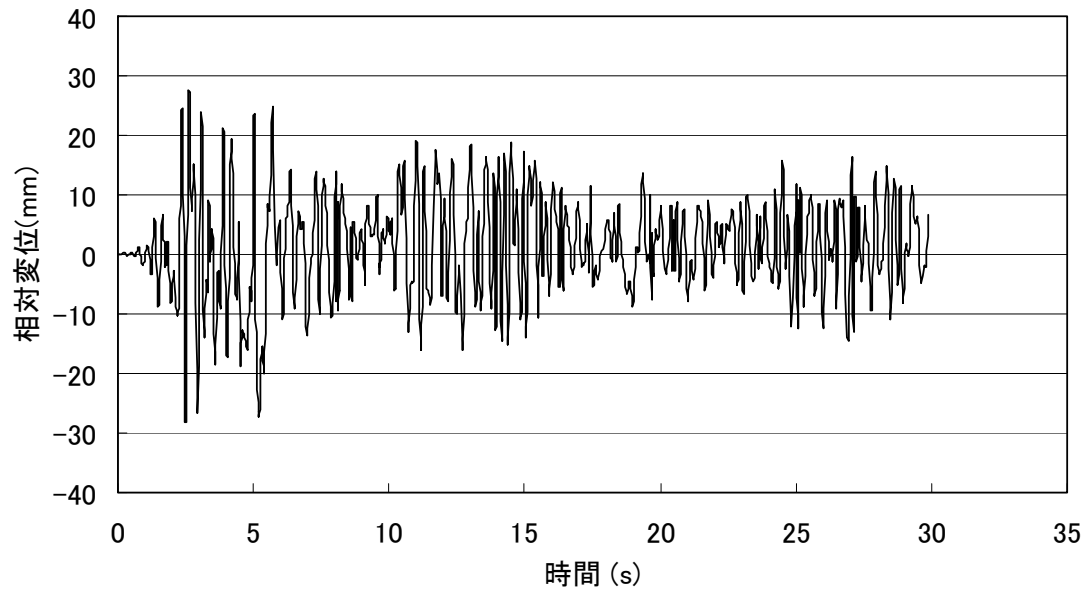
図 3.12 内壁頂部－外壁頂部間の水平方向相対変位時刻歴 (最大相対変位 28.3mm、時刻 2.49s)
