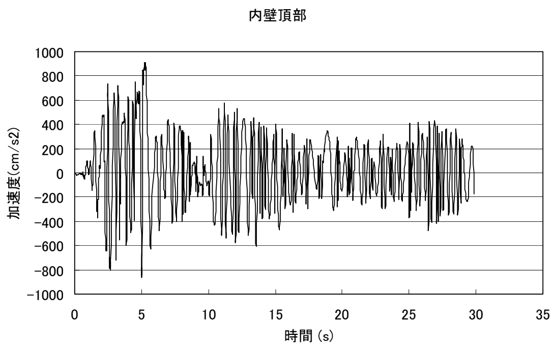
図 3.11 内壁頂部の水平方向加速度時刻歴 (最大加速度 883gal、時刻 5.31s)
