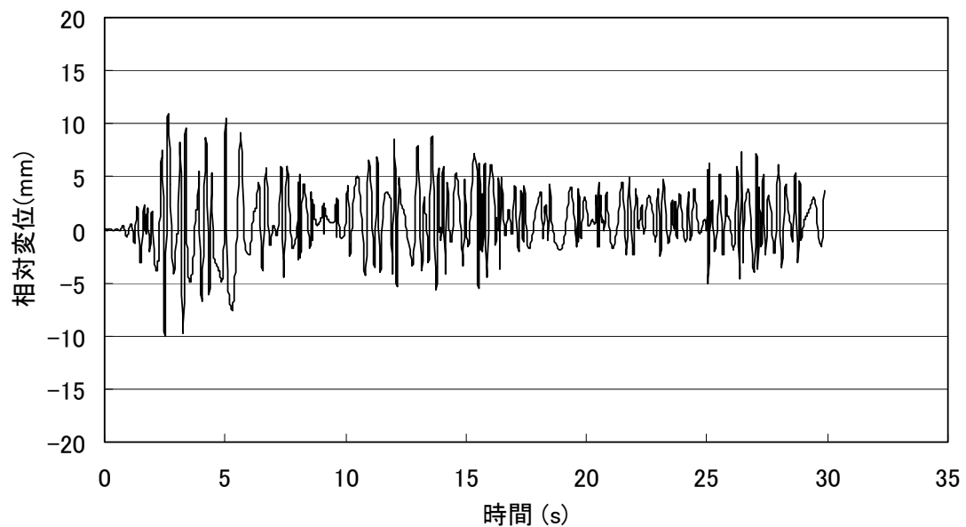
図 3.13 内壁2F部－外壁2F部間の水平方向相対変位時刻歴 (最大相対変位 10.63mm、時刻 2.65s)
