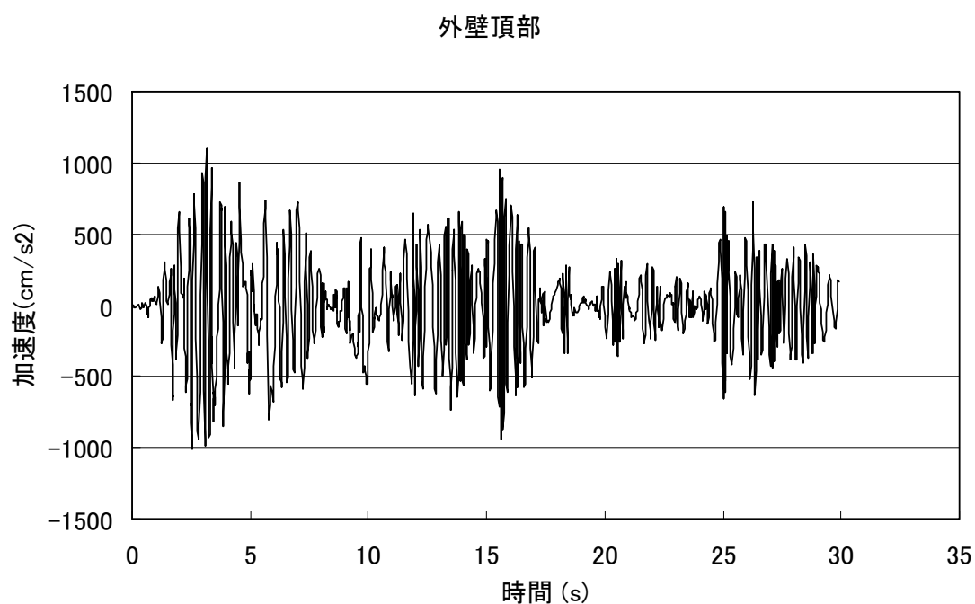
図 3.9 外壁頂部の水平方向加速度時刻歴 (最大加速度 1098gal、時刻 3.14s)
