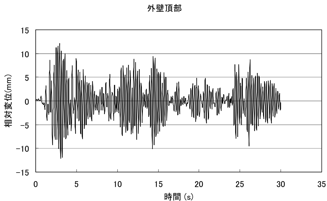
図 3.8 外壁頂部スラブ間の水平方向相対変位時刻歴 (最大相対変位 12.2mm、時刻 2.93s)
