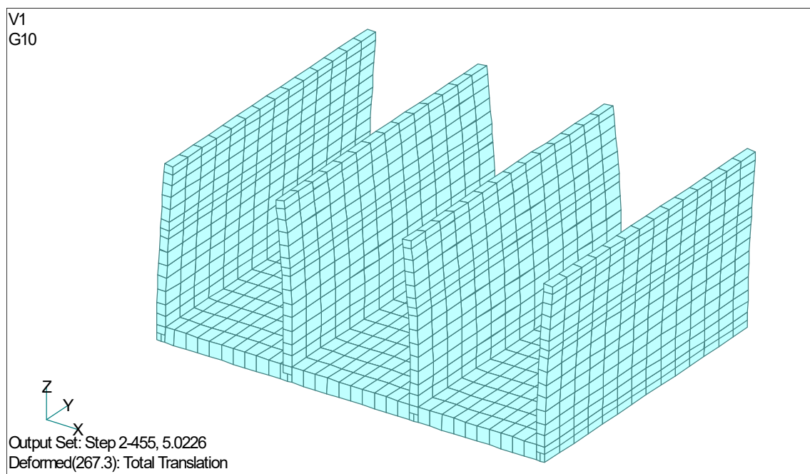
図 3.15 内壁頂部ースラブ間の水平方向最大相対変位発生時刻の変形図 (最大相対変位 26.4mm、時刻 5.02s)
