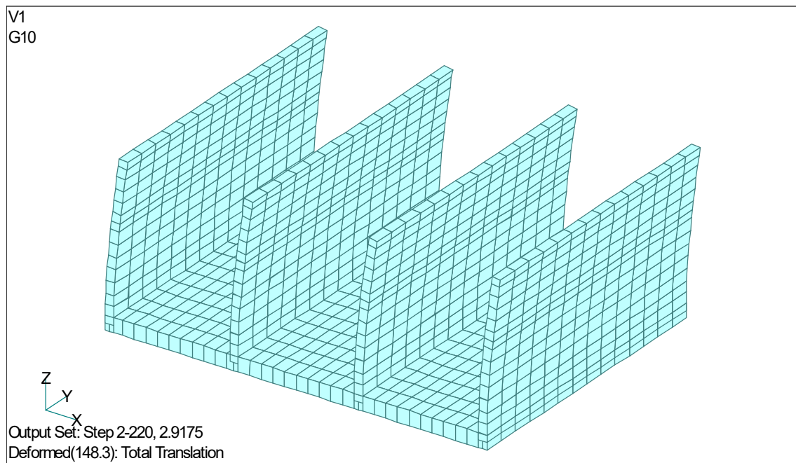
図 3.14 外壁頂部ースラブ間の水平方向最大相対変位発生時刻の変形図 (最大相対変位 12.2mm、時刻 2.93s)
