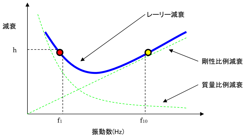
図 2.30 レーリー減衰
