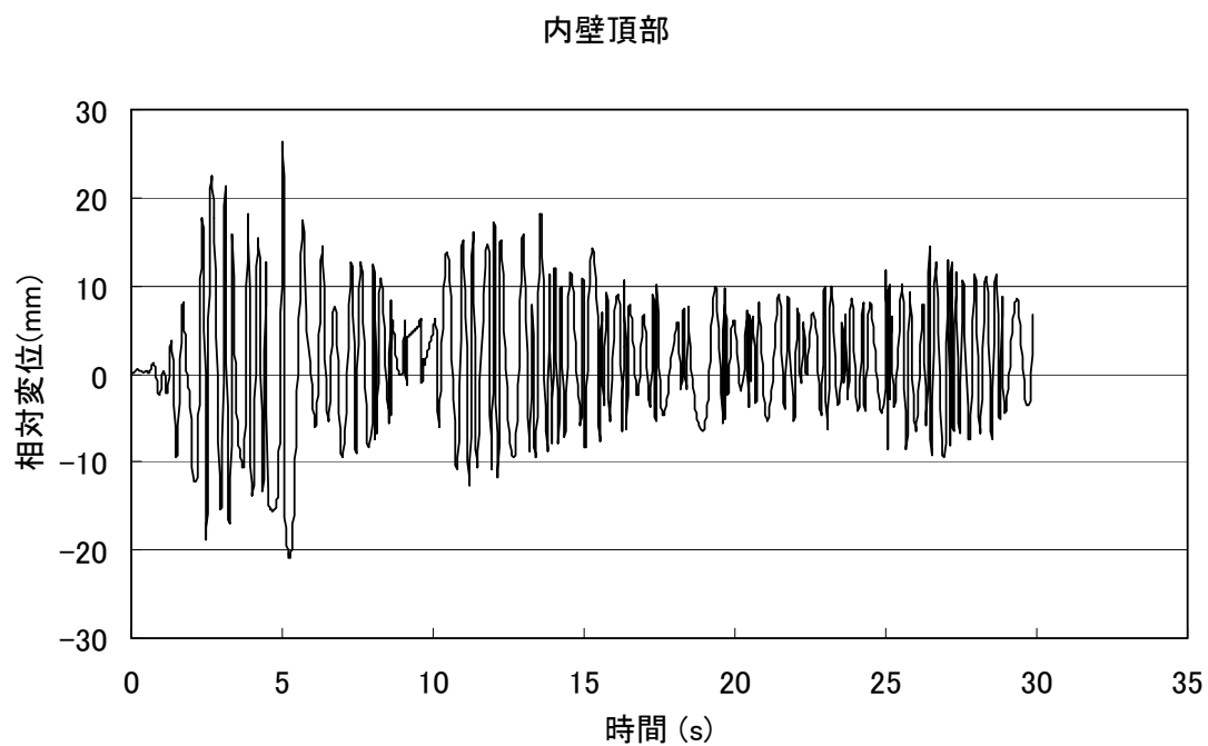
図 3.10 内壁頂部—スラブ間の水平方向相対変位時刻歴 (最大相対変位 26.4mm、時刻 5.02s)
