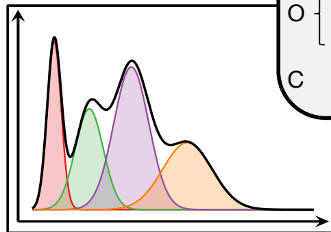
UV-Vis Spectra
