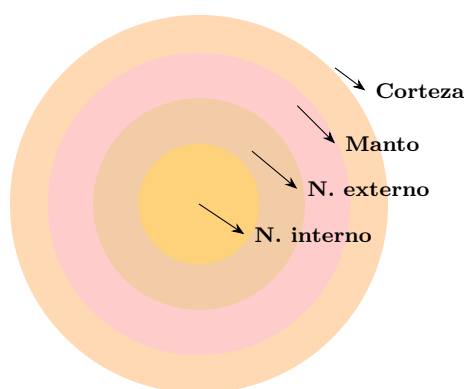
Capas internas de la Tierra
