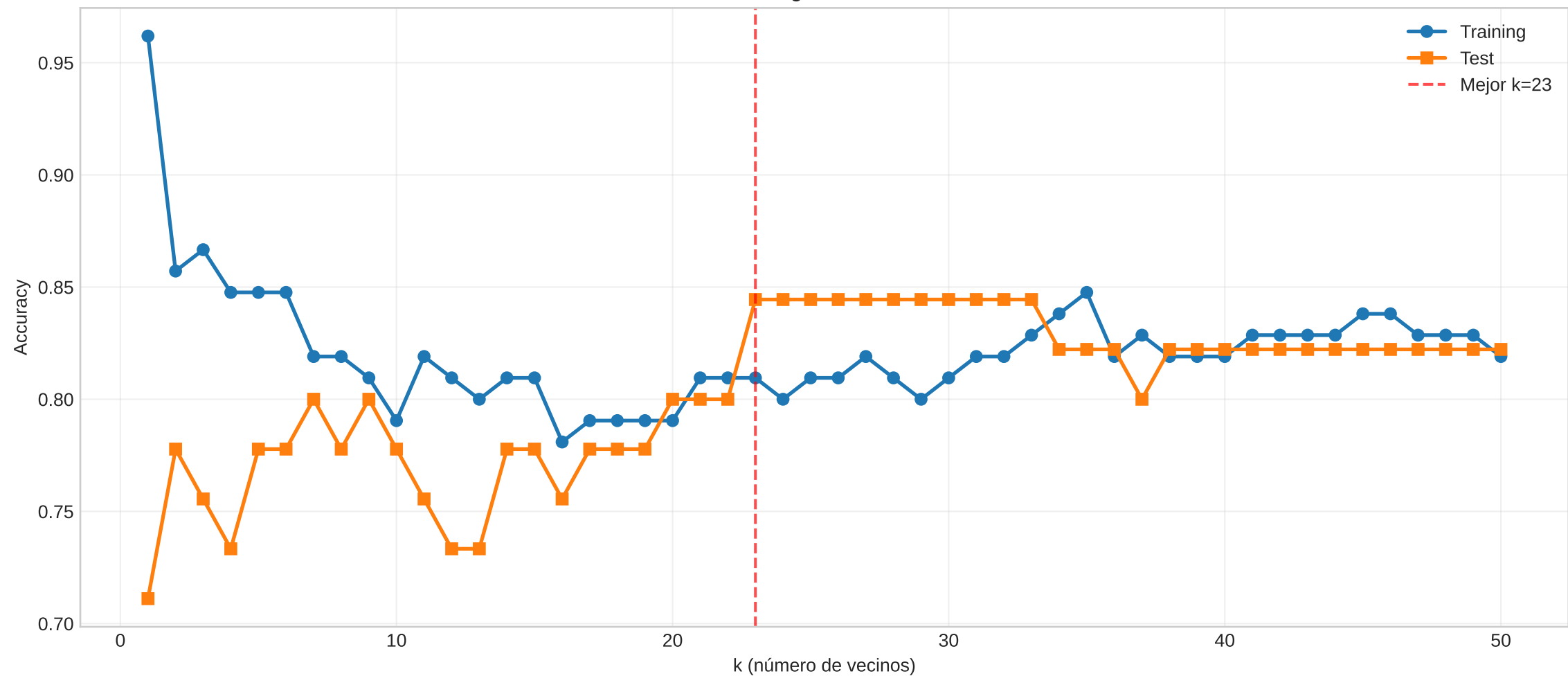
Trade-off Sesgo-Varianza en KNN
