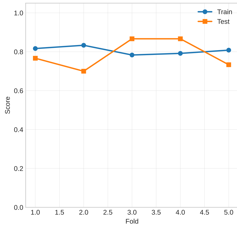
F1
