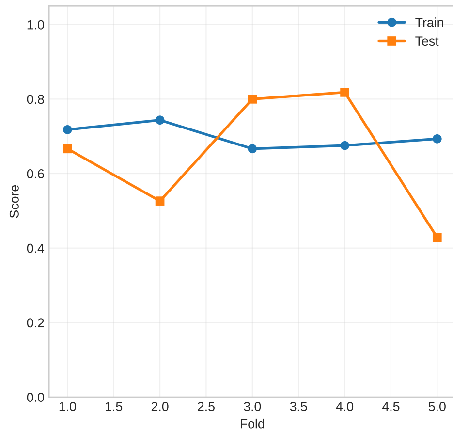
F1
