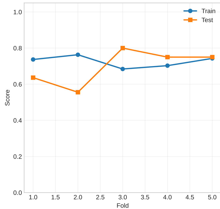
ROC_AUC
