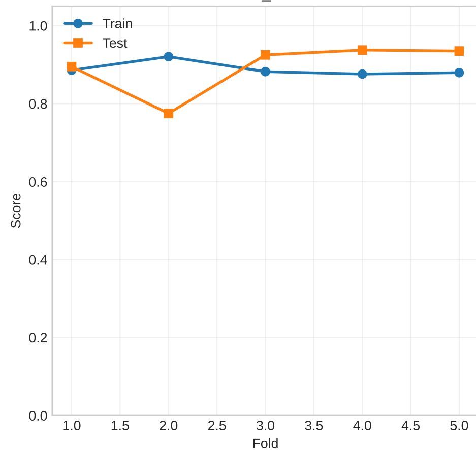
ROC_AUC
