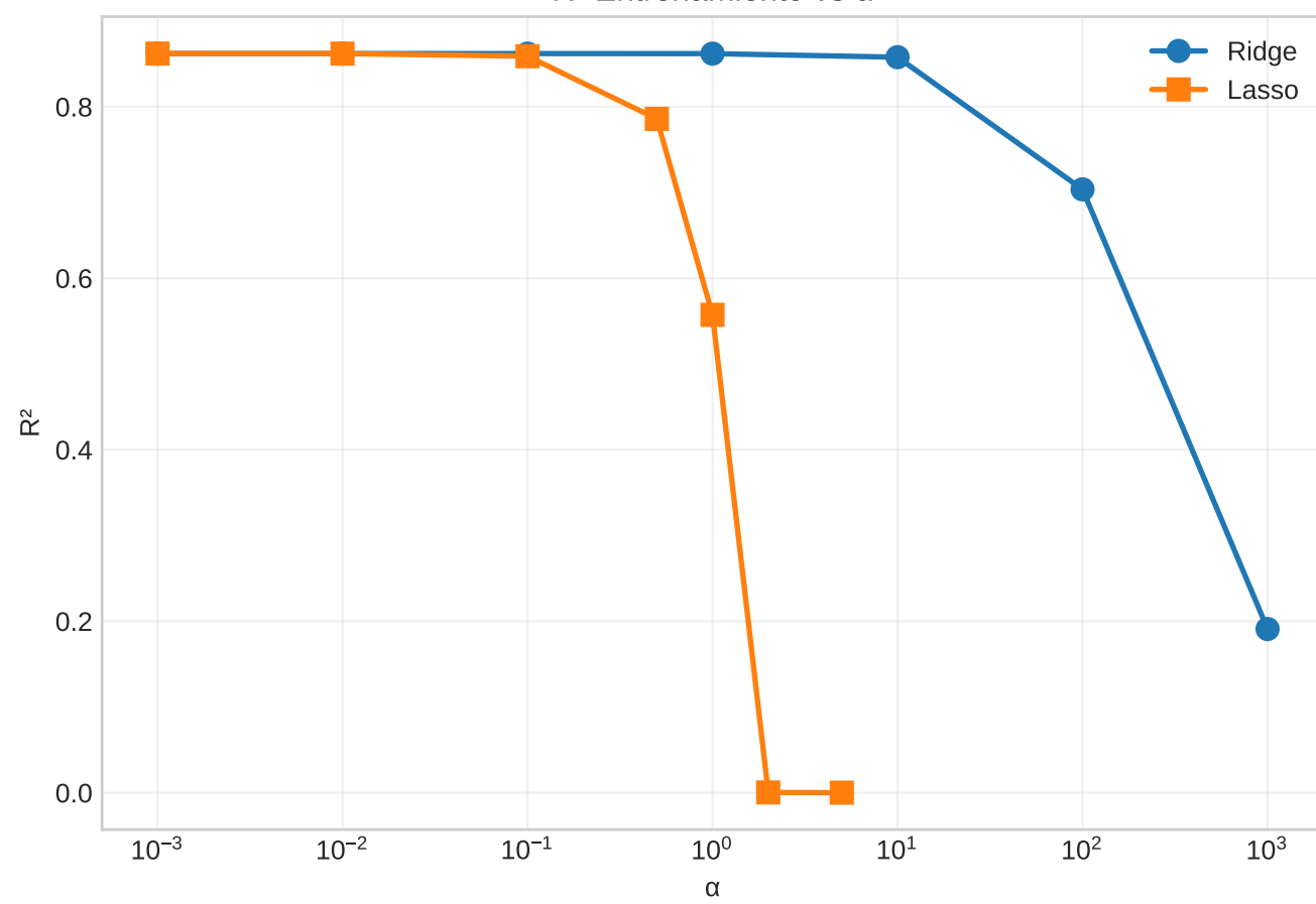
R^2 Entrenamiento vs \alpha
