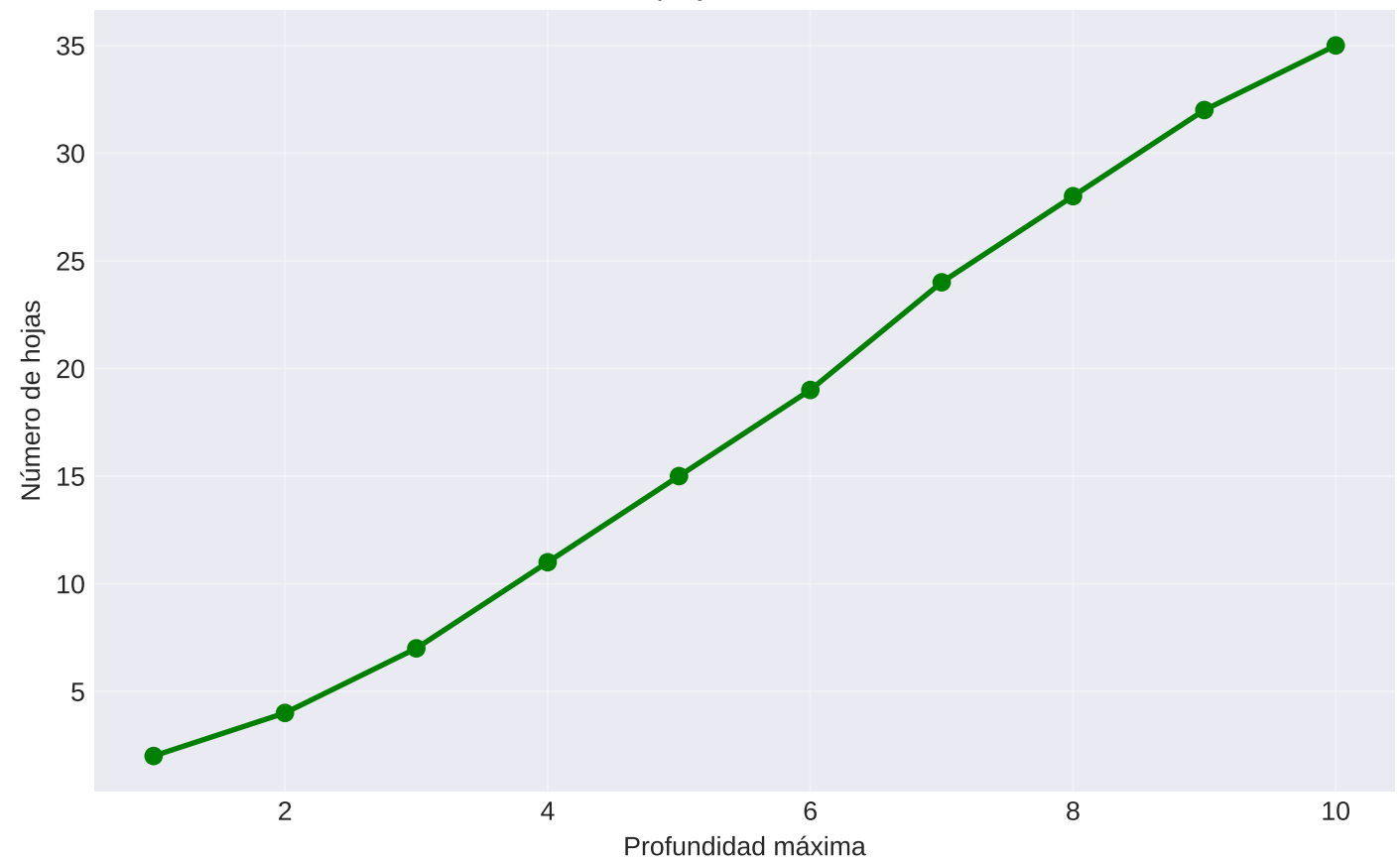
Complejidad del Árbol
