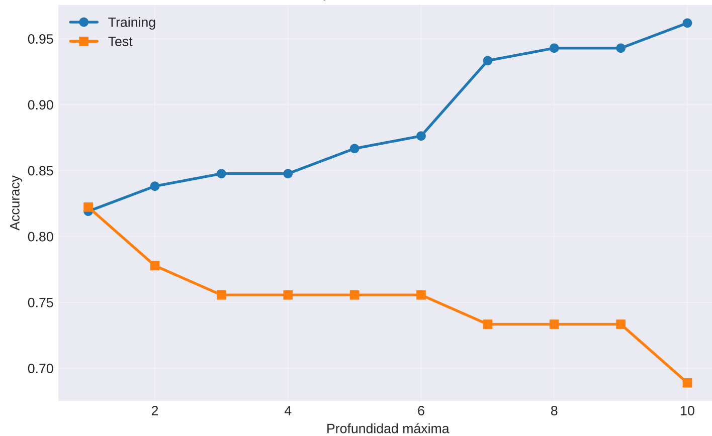
Accuracy vs Profundidad del Árbol
