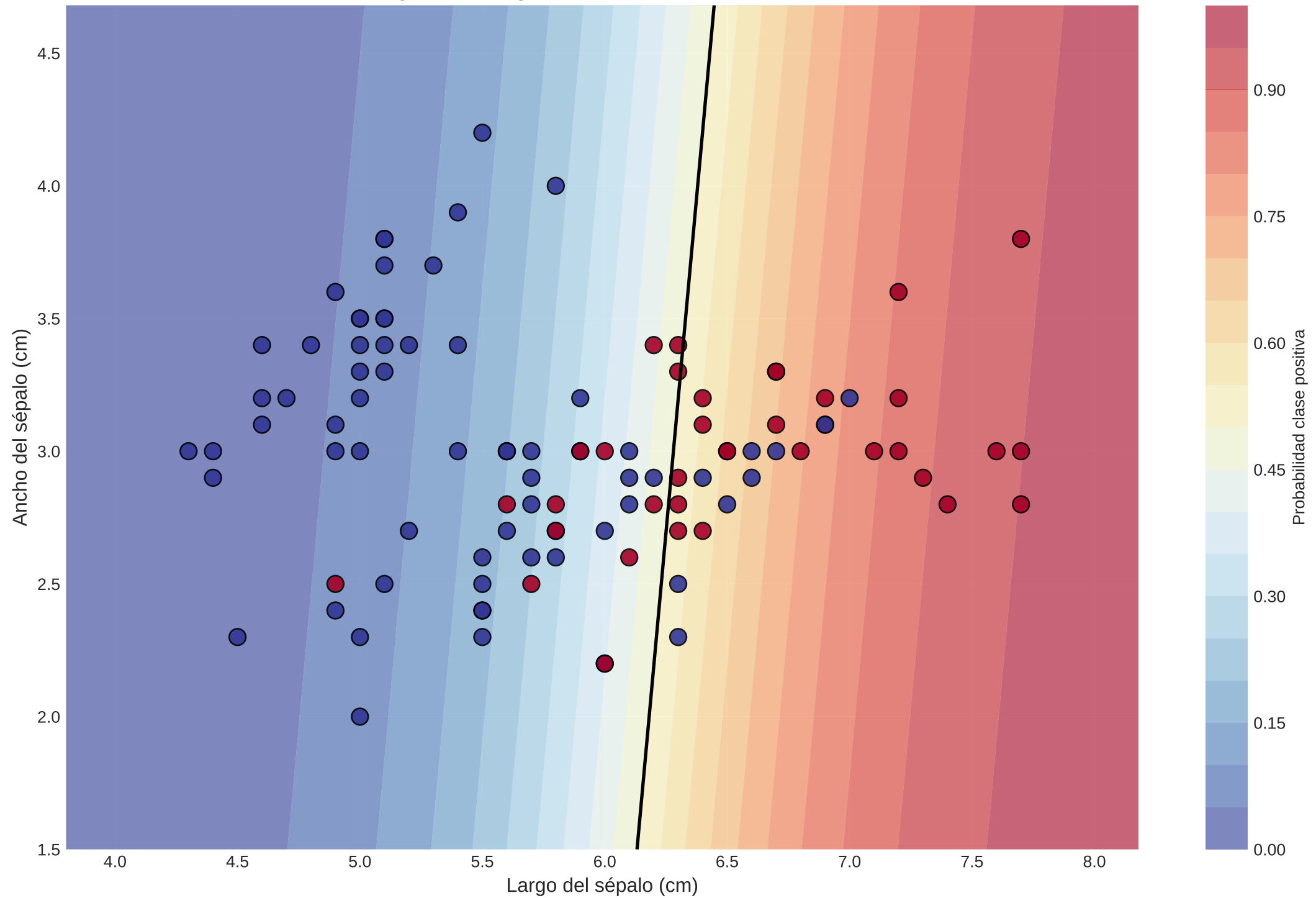
Regresión Logística - Frontera de Decisión
