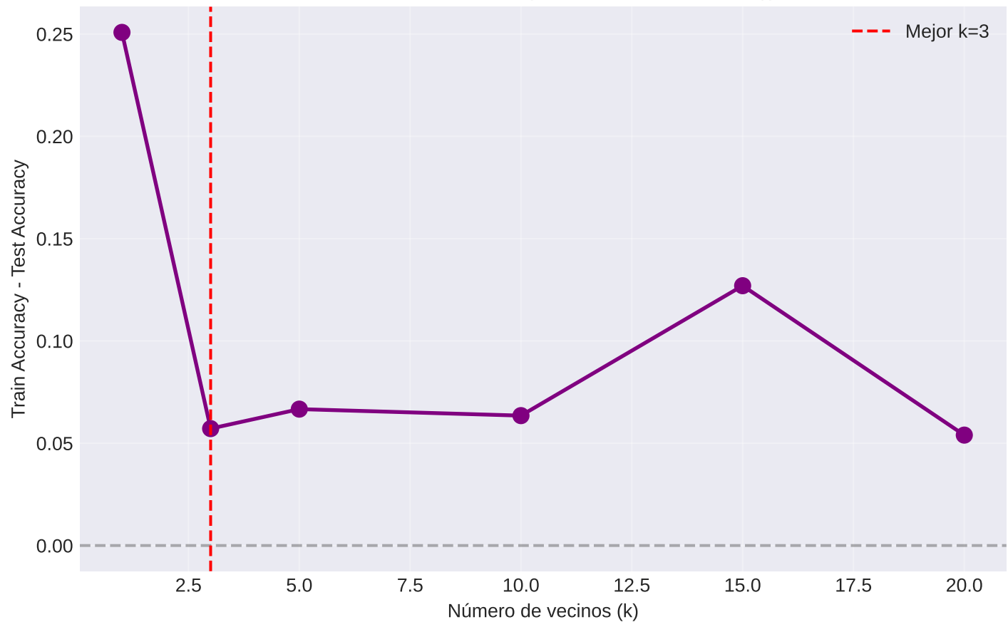
Diferencia Train-Test (Indicador de Overfitting)
