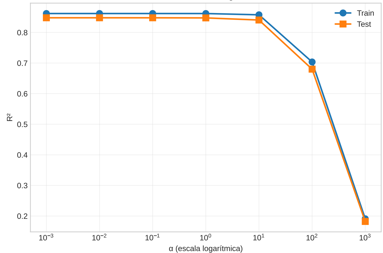
R^2 vs Parámetro de Regularización
