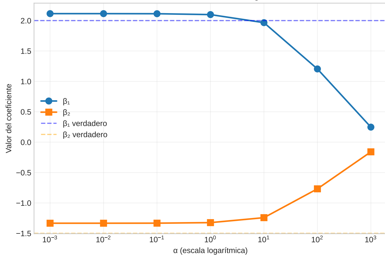
Coeficientes vs Parámetro de Regularización
